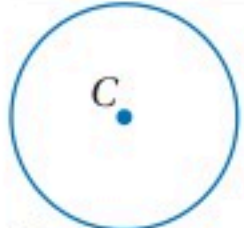
الدائرة C أو \odot C
