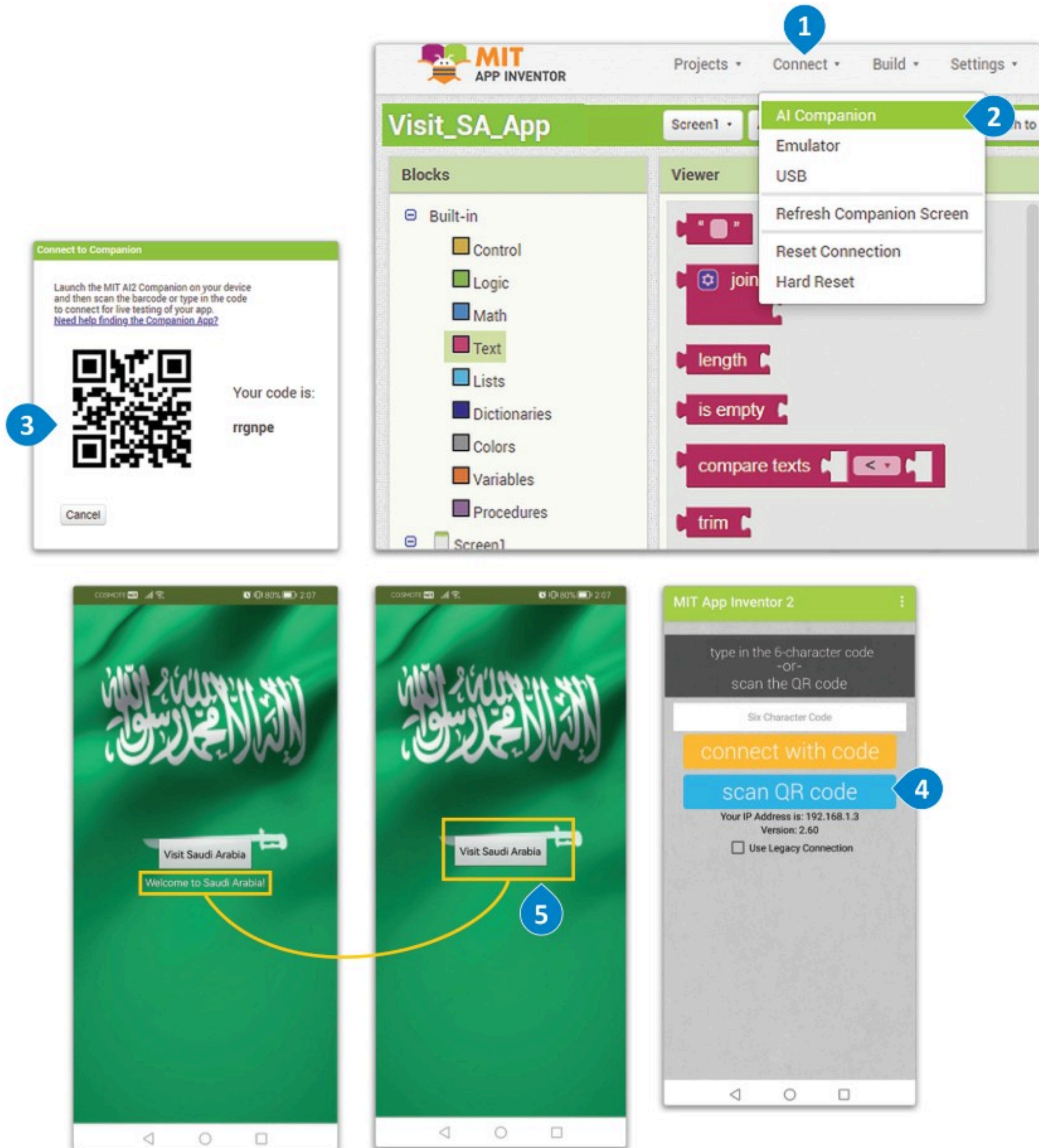
شكل 3.16: اختبار التطبيق باستخدام MIT AI2 Companion
