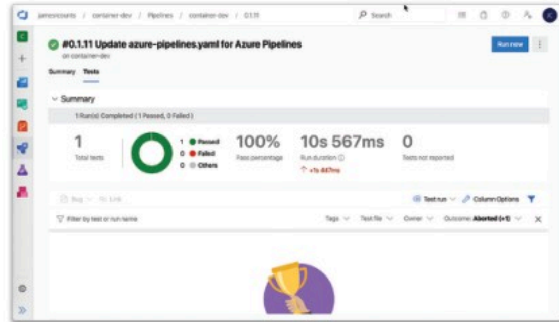
شكل 1.18: نشر البرنامج
