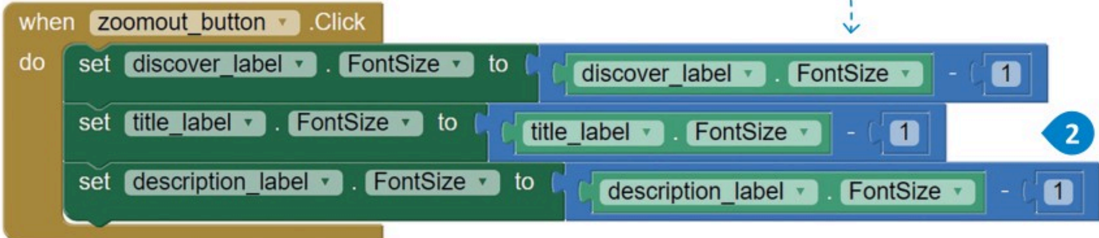
شكل 4.9: برمجة زر التصغير
