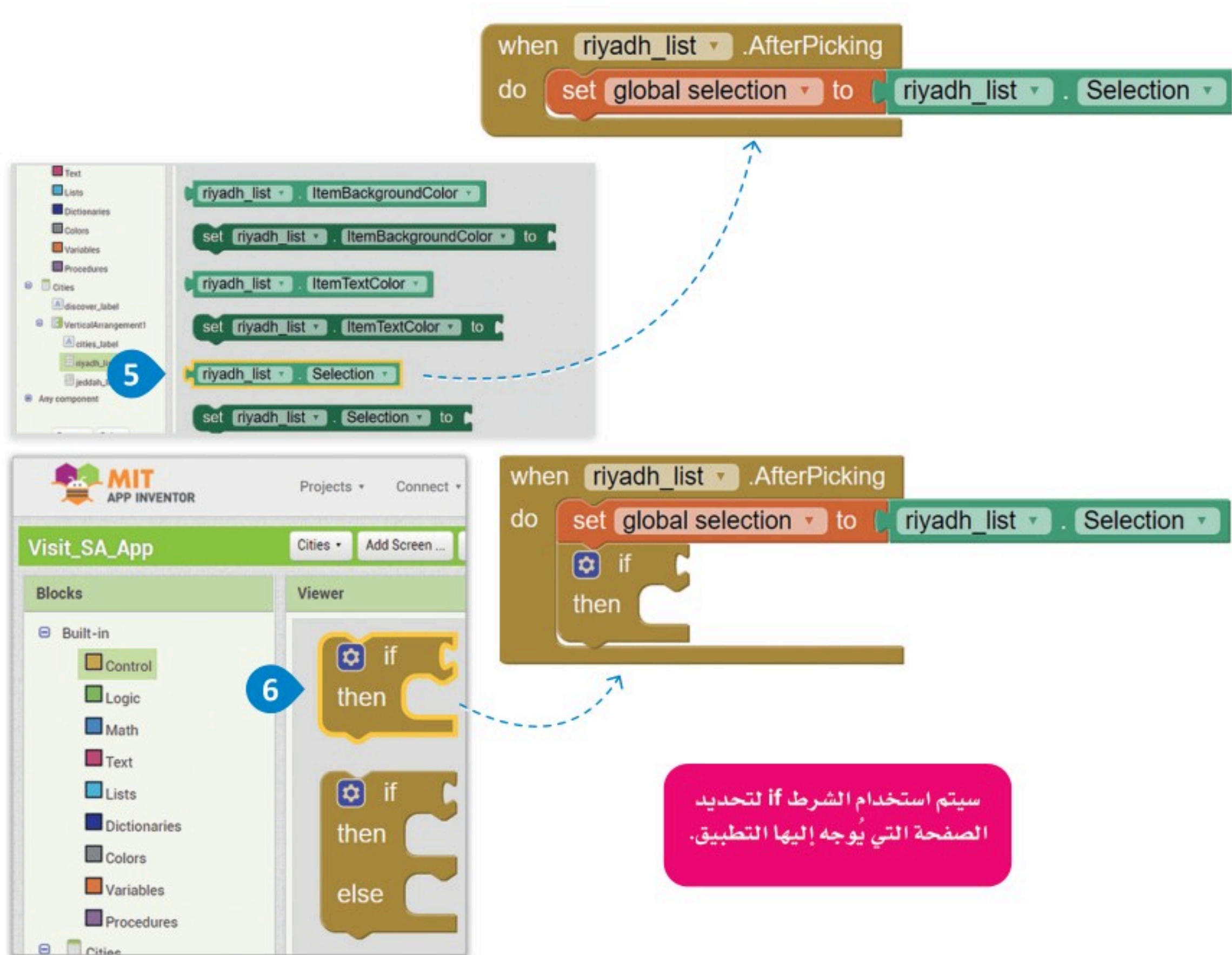
شكل 3.39: تحديد الصفحة من ListPicker (قائمة الخيارات)
