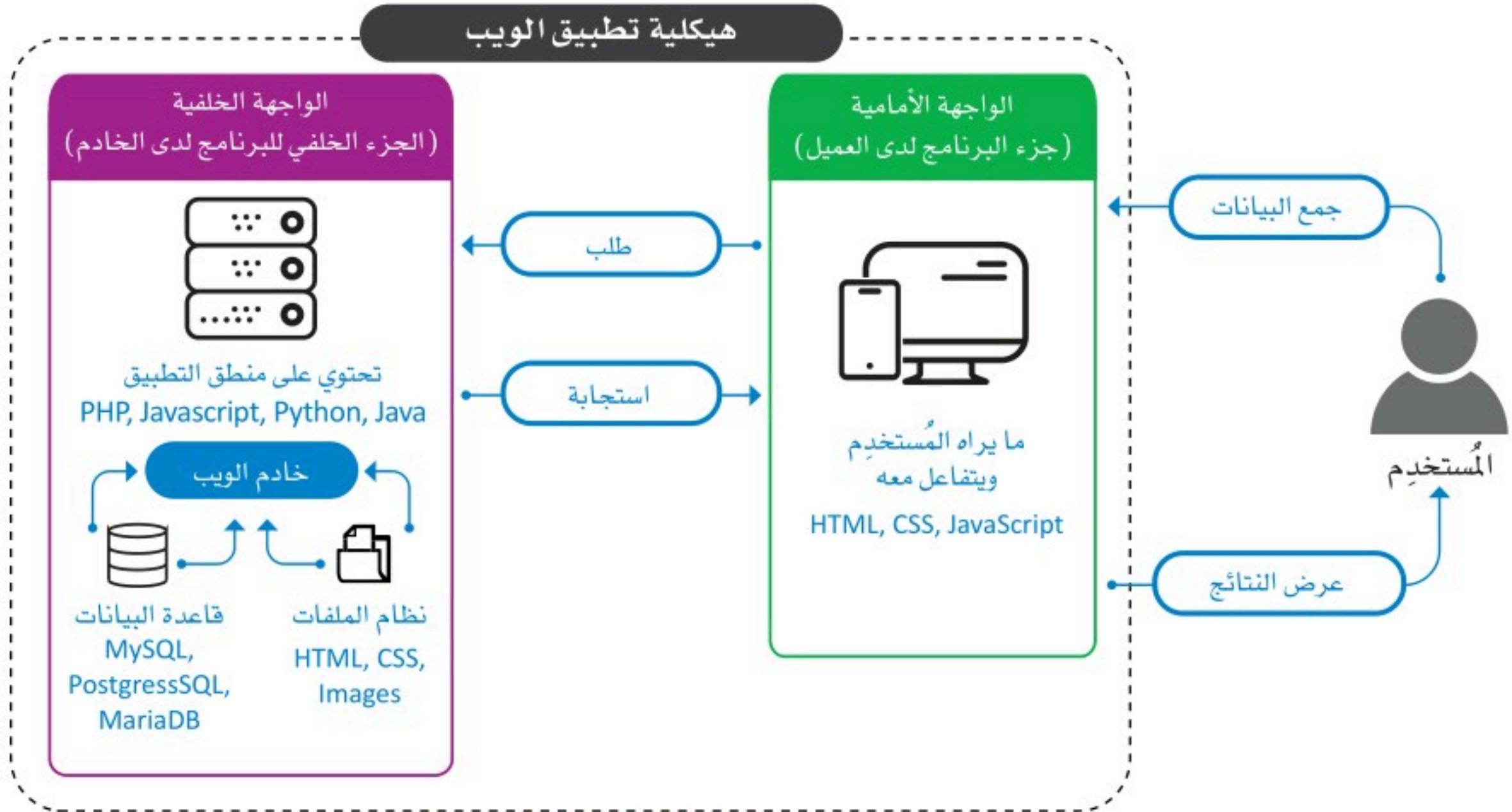
شكل 1.20: الهيكلية الأساسية لتطبيق الويب
