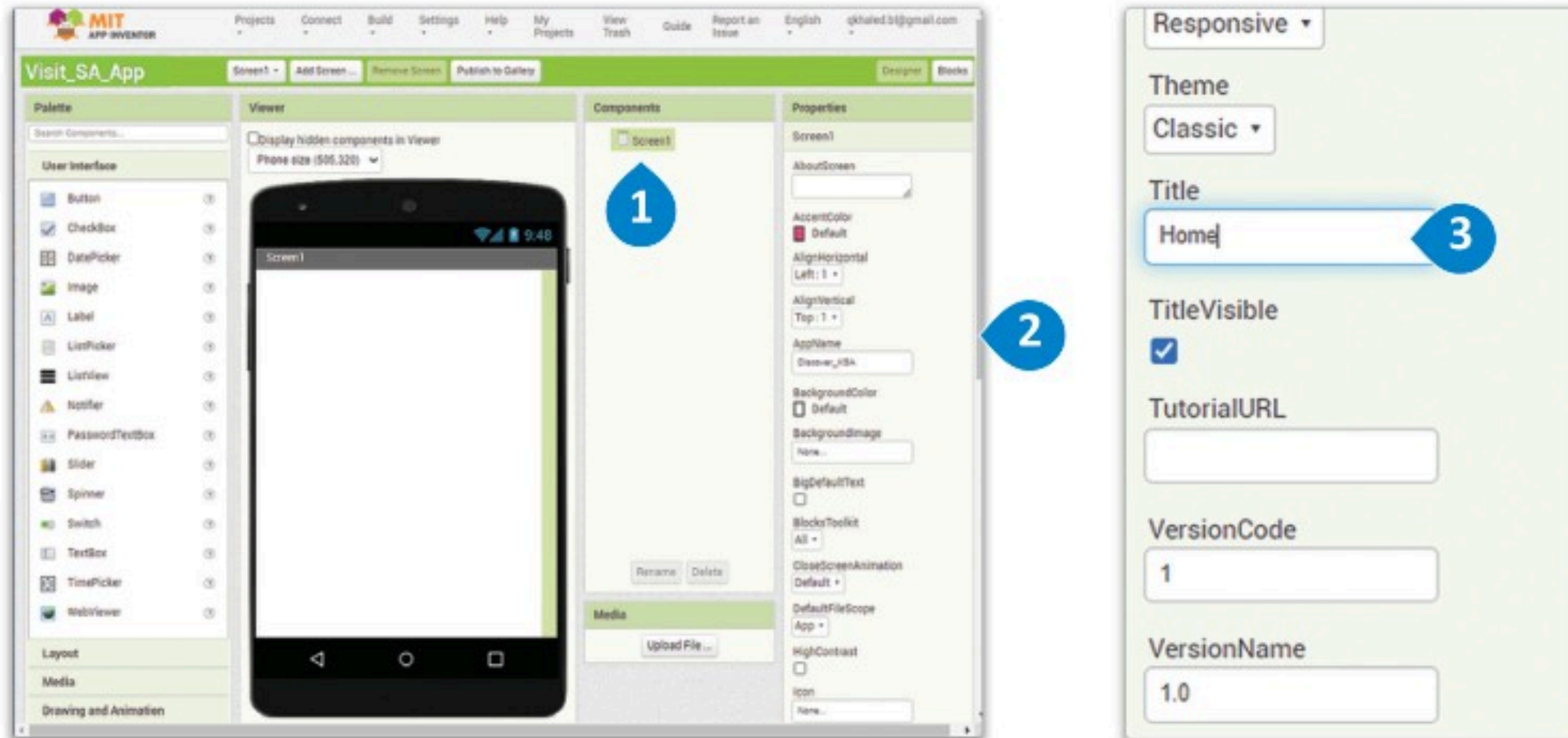
شكل 3.5: تغيير عنوان الشاشة
