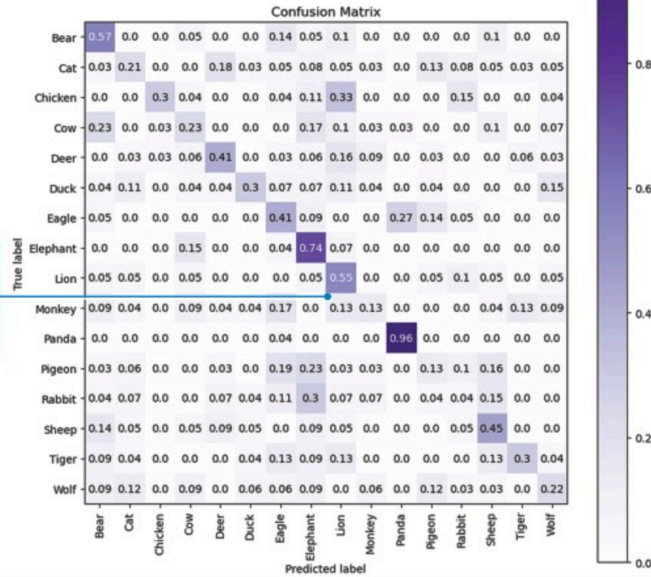
شكل 4.7: مصفوفة الدقة الخاصة بأداء خوارزمية MultinomialNB
