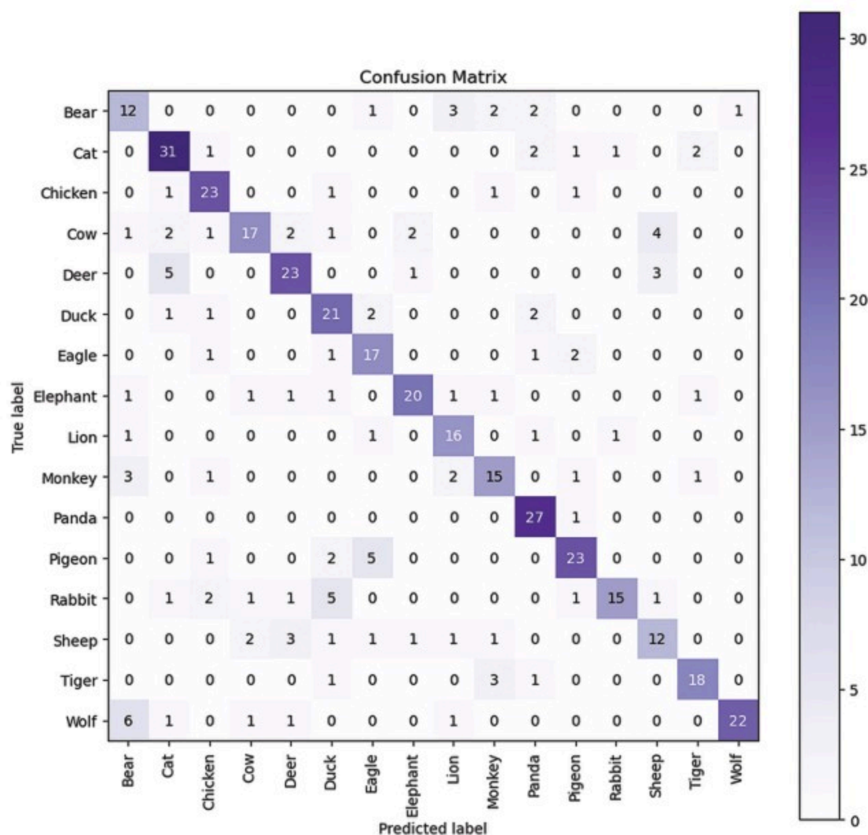
شكل 4.11: مصفوفة الدقة لأداء خوارزمية SGDClassifier
