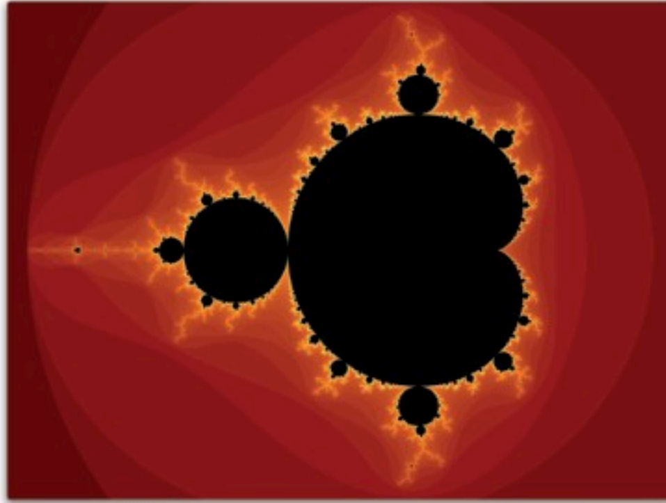
شكل 4.25: فراكتل ماندلبروت
