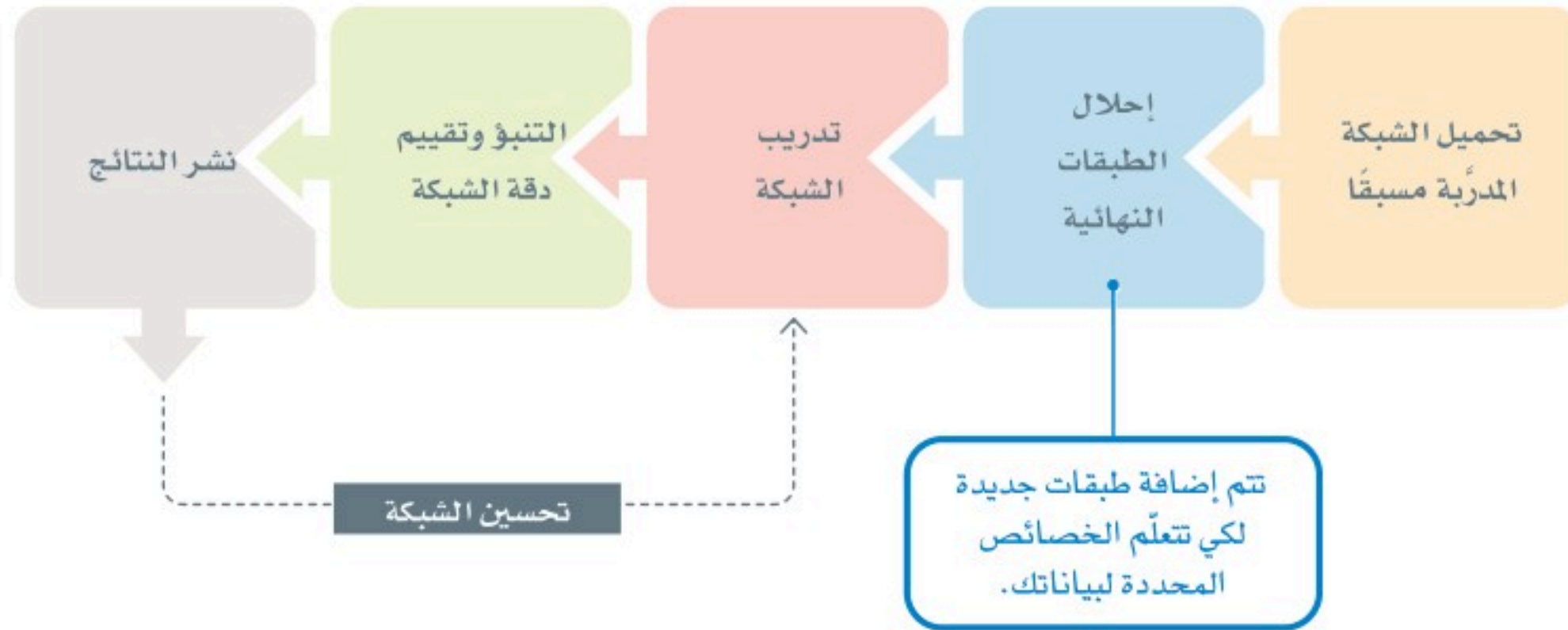
شكل 4.15: إعادة استخدام الشبكة المدربة مسبقاً
