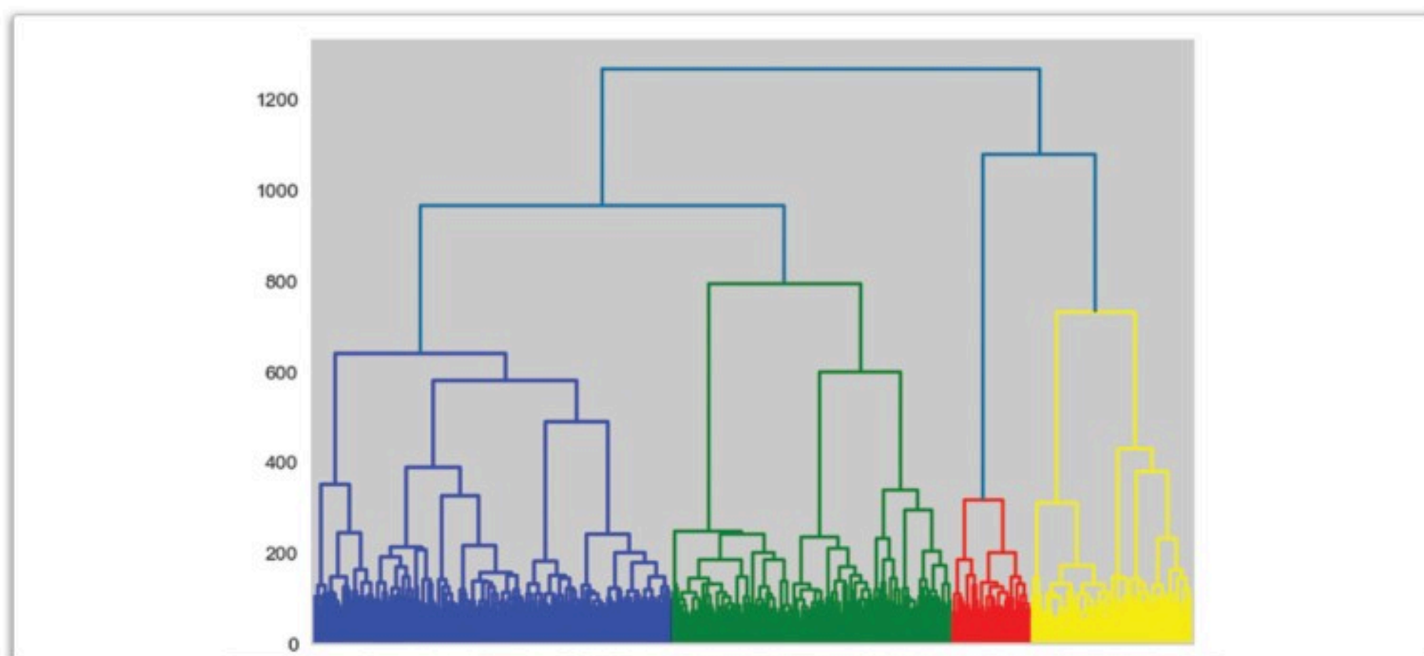
شكل 4.24: الرسم الشجري الهرمي لفئات وجوه الحيوانات المختلفة باستخدام نموذج VGG16
