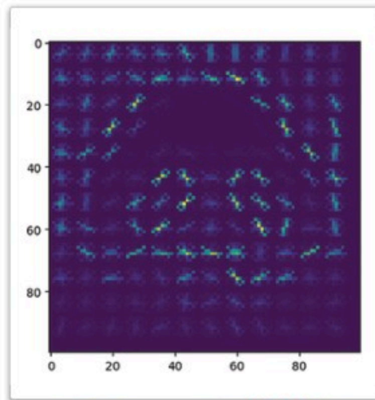
شكل 4.10: مخطط تكراري للتدرجات الموجهة لصورة
