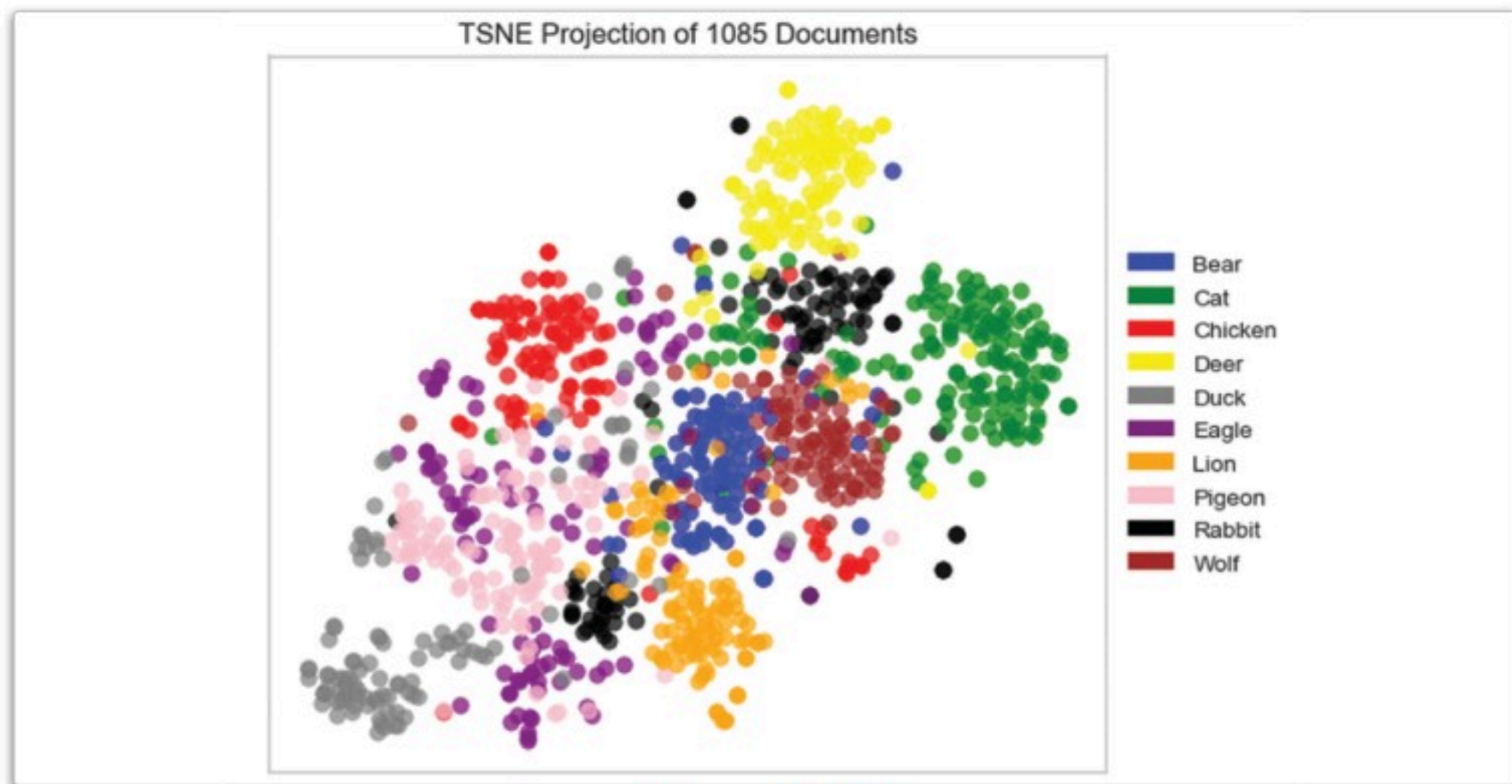
شكل 4.20: تصوير العناقيد
