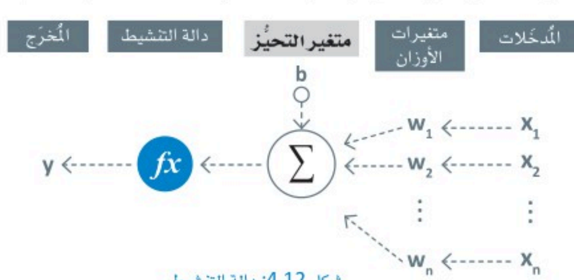
شكل 4.12: دالة التنشيط
