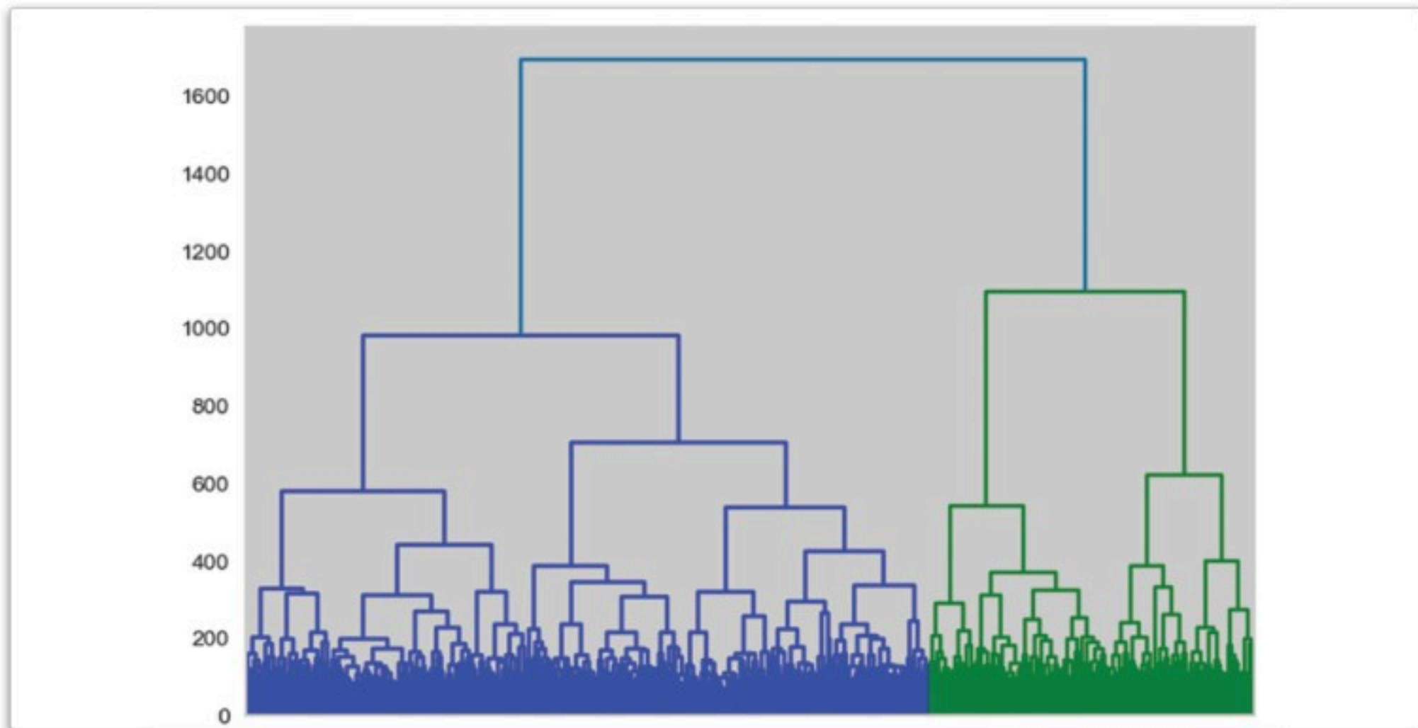
شكل 4.19: الرسم الشجري يُصنف البيانات إلى عنقودين
