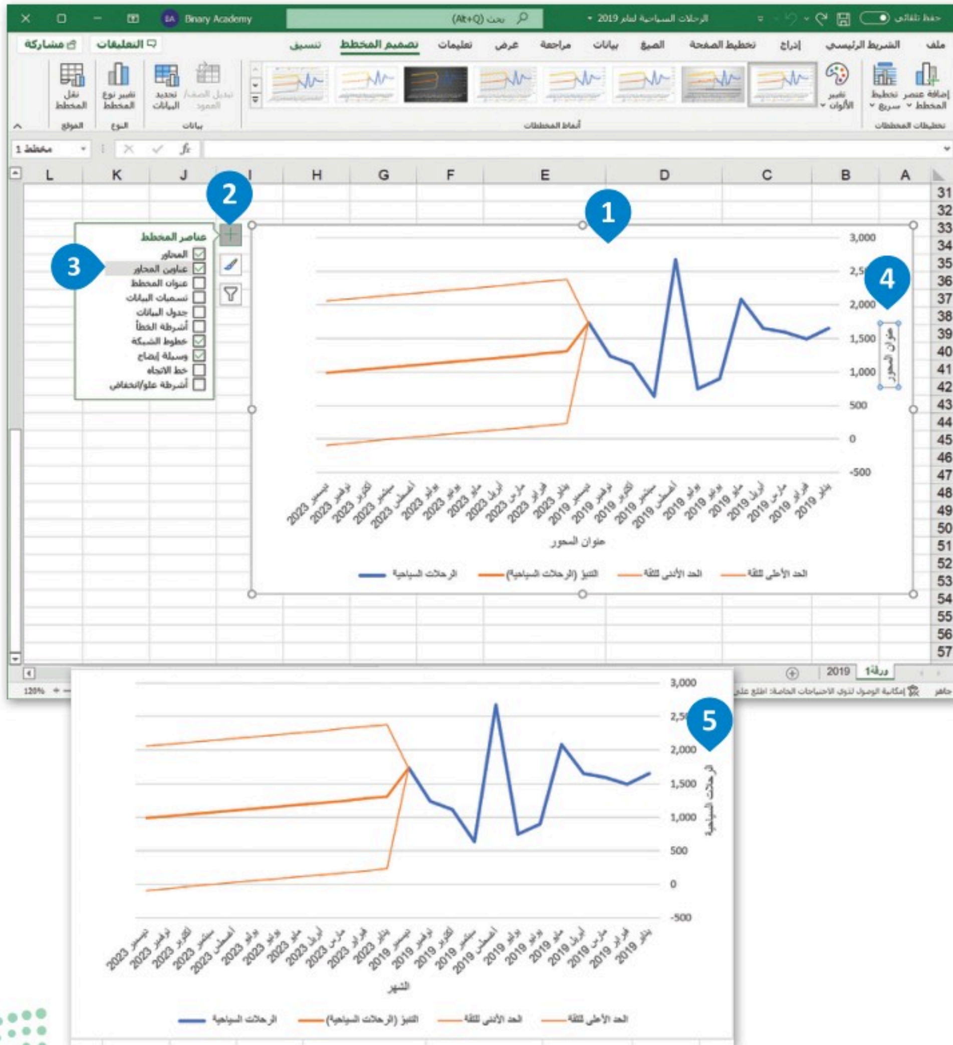
شكل 4.17: تغيير عناوين التسمية
