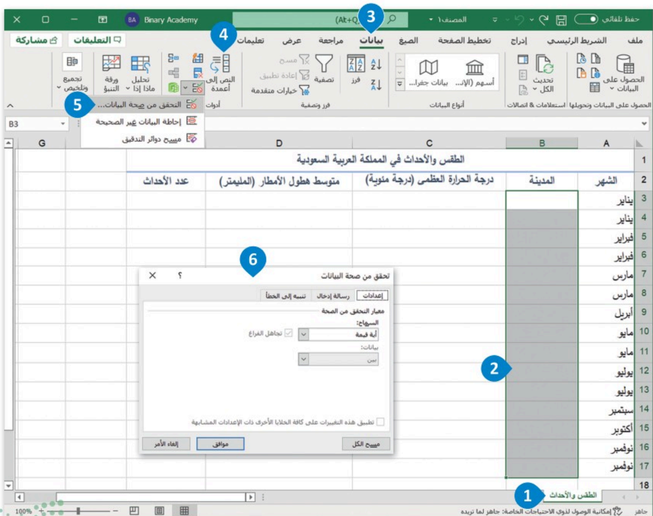
الشكل 2.28: بدء عملية التحقق من صحة البيانات
