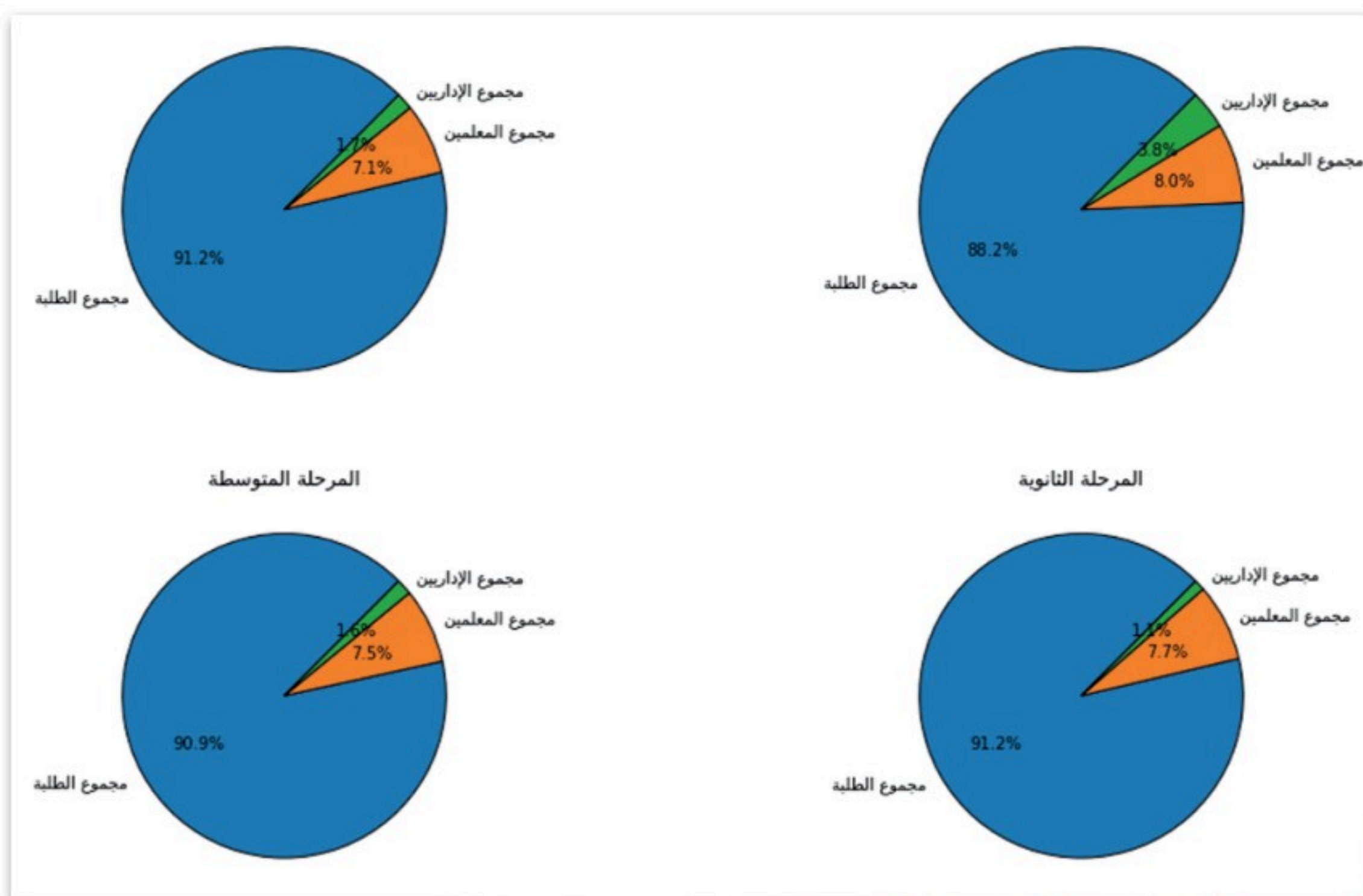
الشكل 3.54: المخطط الدائري
