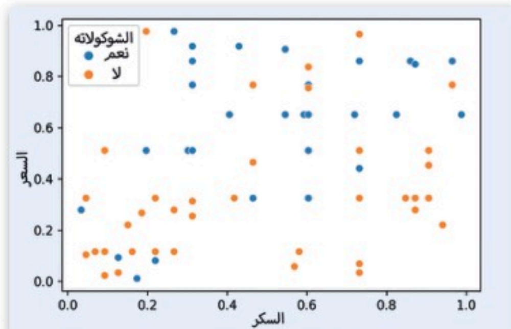
الشكل 3.5: التحليل الرسومي متعدد المتغيرات
