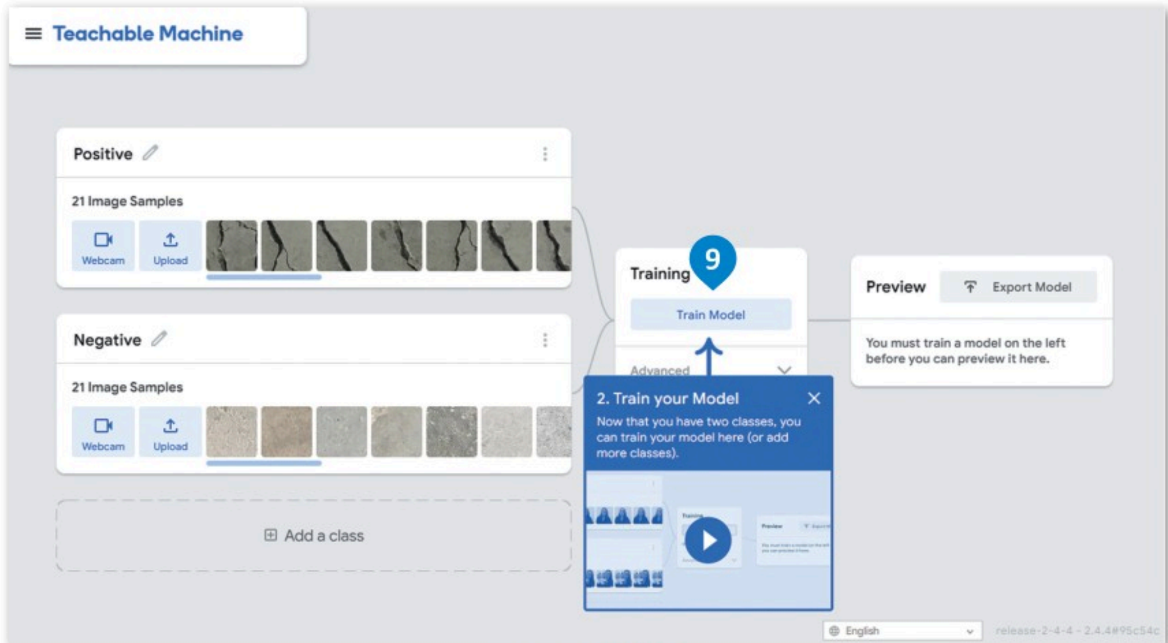
شكل 4.5: إنشاء نموذج وتدريبه
