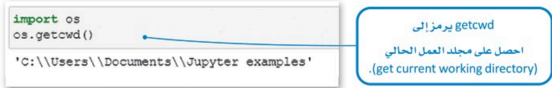
الشكل 3.14: مكتبة نظام التشغيل
