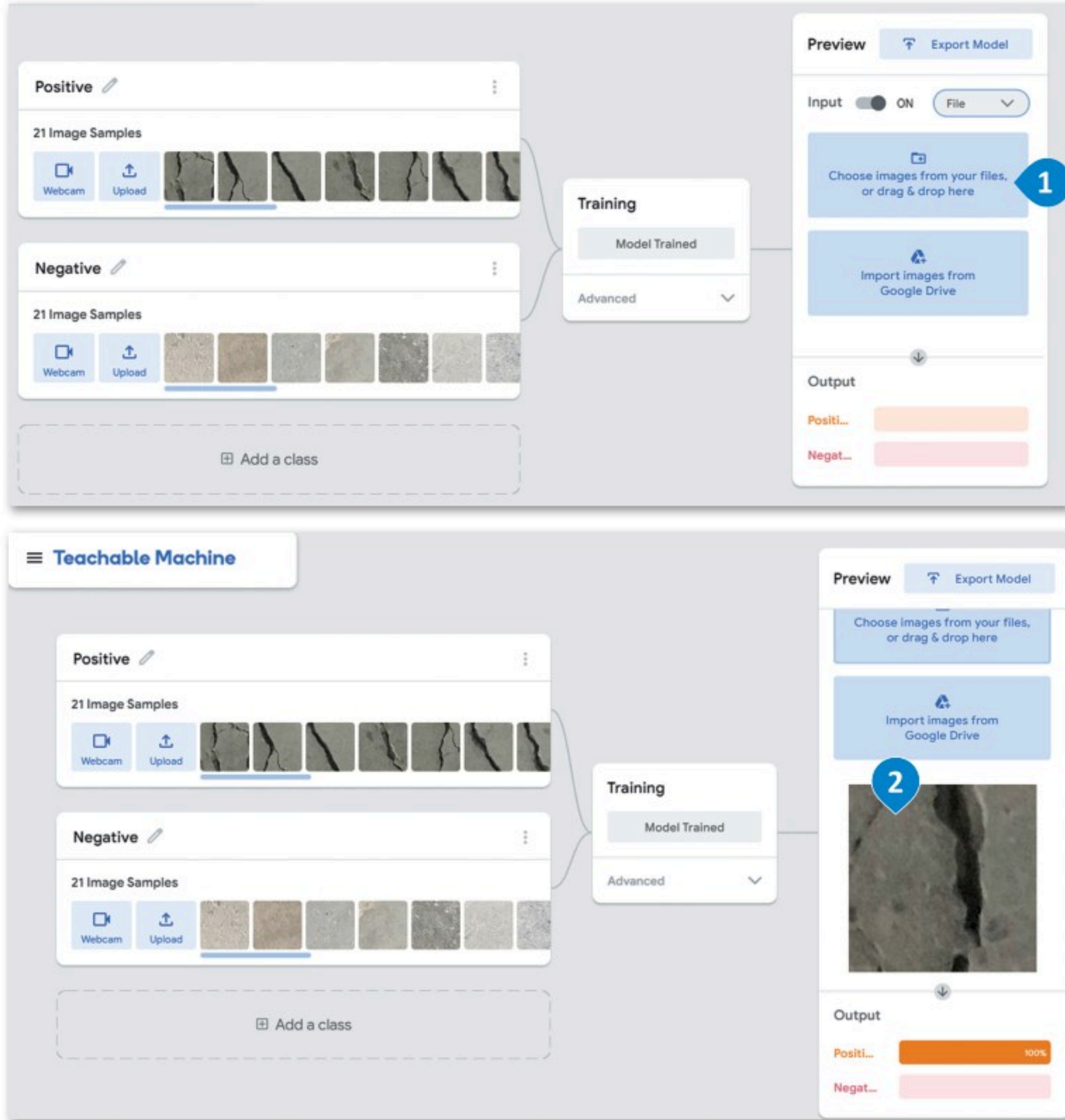
شكل 4.6: اختبار وتقييم نموذج
