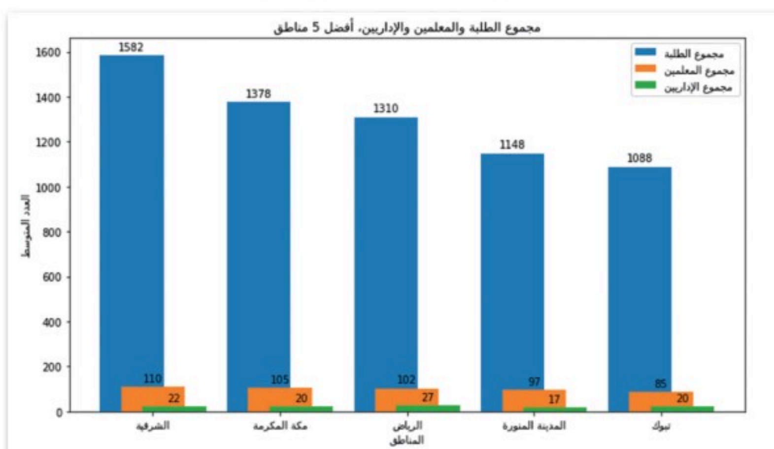
الشكل 3.49: المخطط الشريطي المجمع
