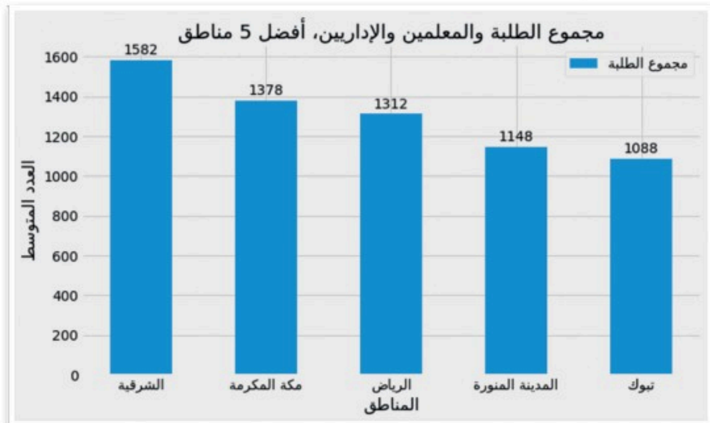
الشكل 3.47: المخطط الشريطي
