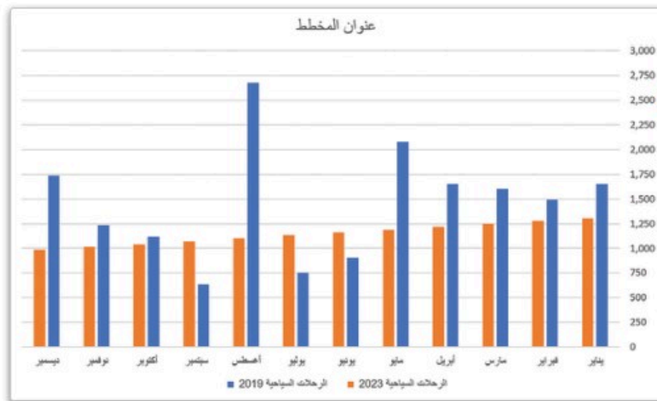
شكل 4.21: مخطط عمودي متفاوت المسافات
