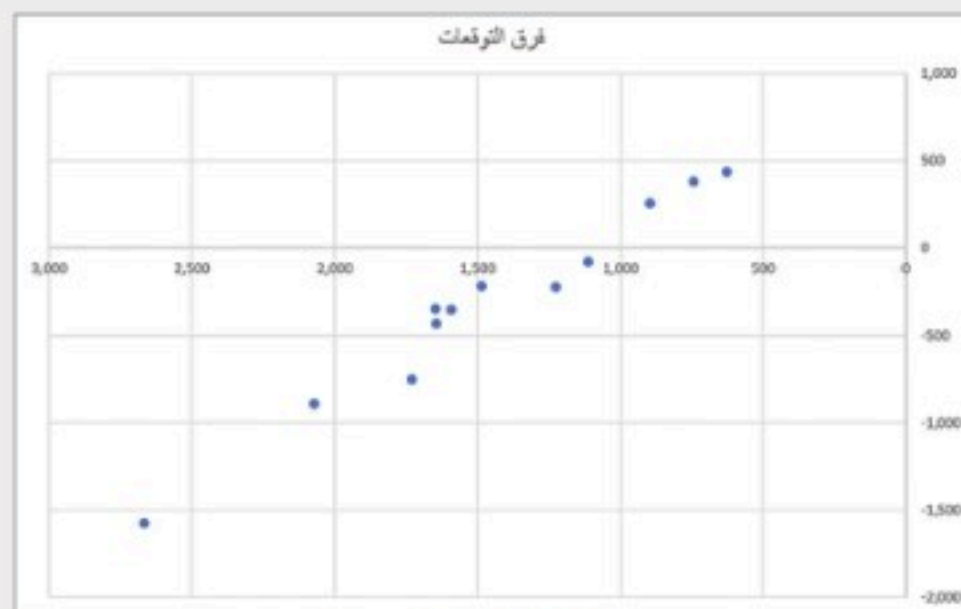
شكل 4.26: مخطط مبعثر
