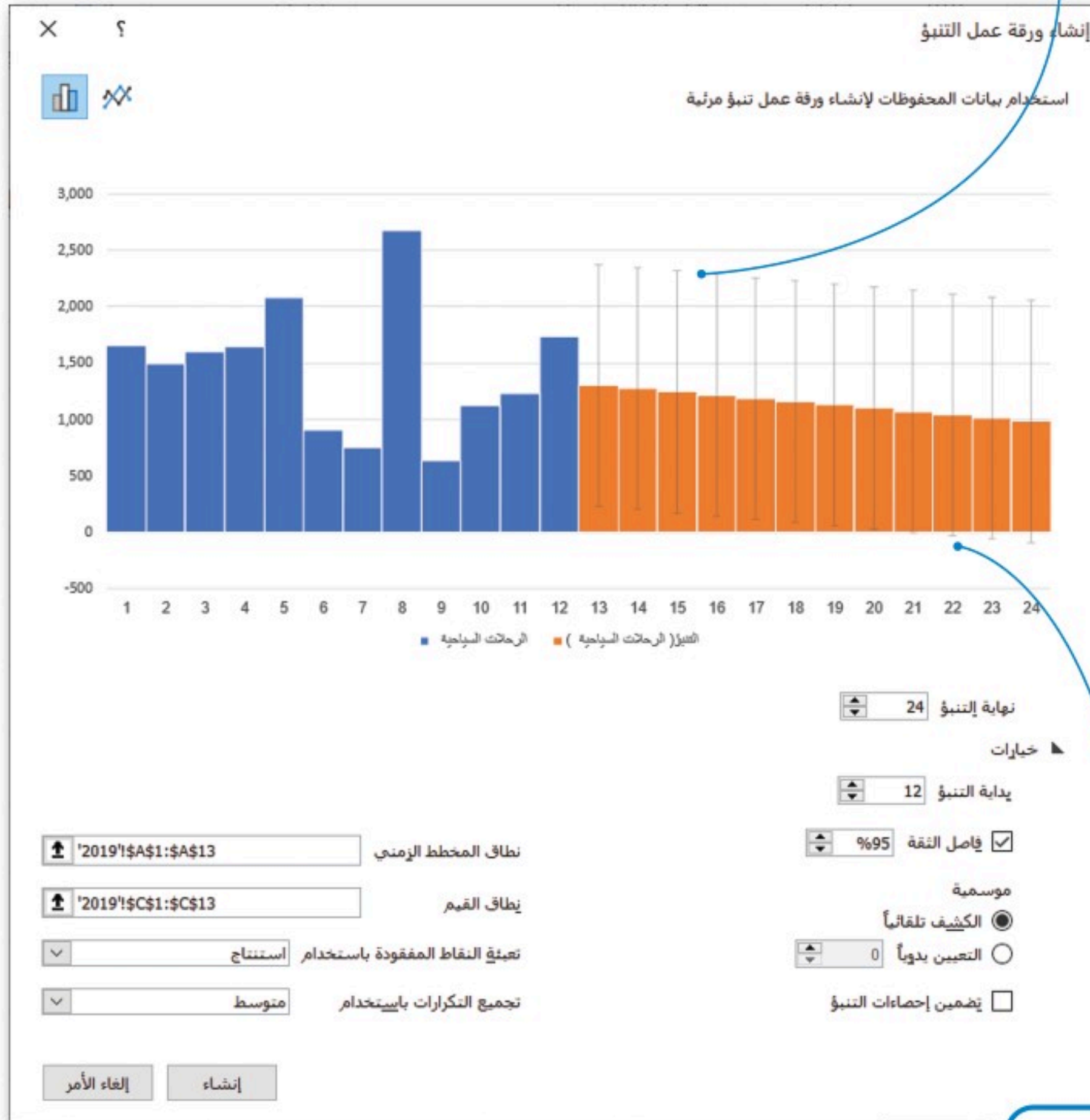
شكل 4.14: المخطط العمودي
