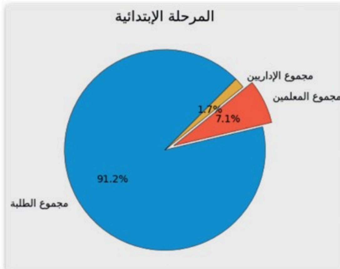
الشكل 3.50: مخطط دائري
