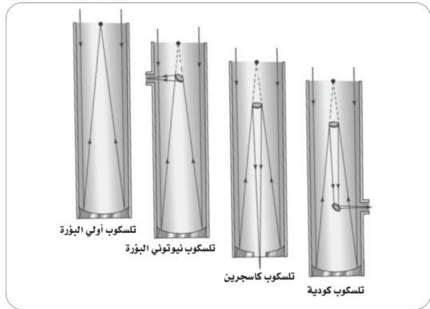
الشكل 9-3 أنواع التلسكوبات العاكسة.
