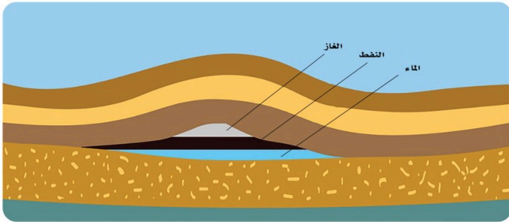
الشكل 3-5 مصائد الطيات المحدبة.
