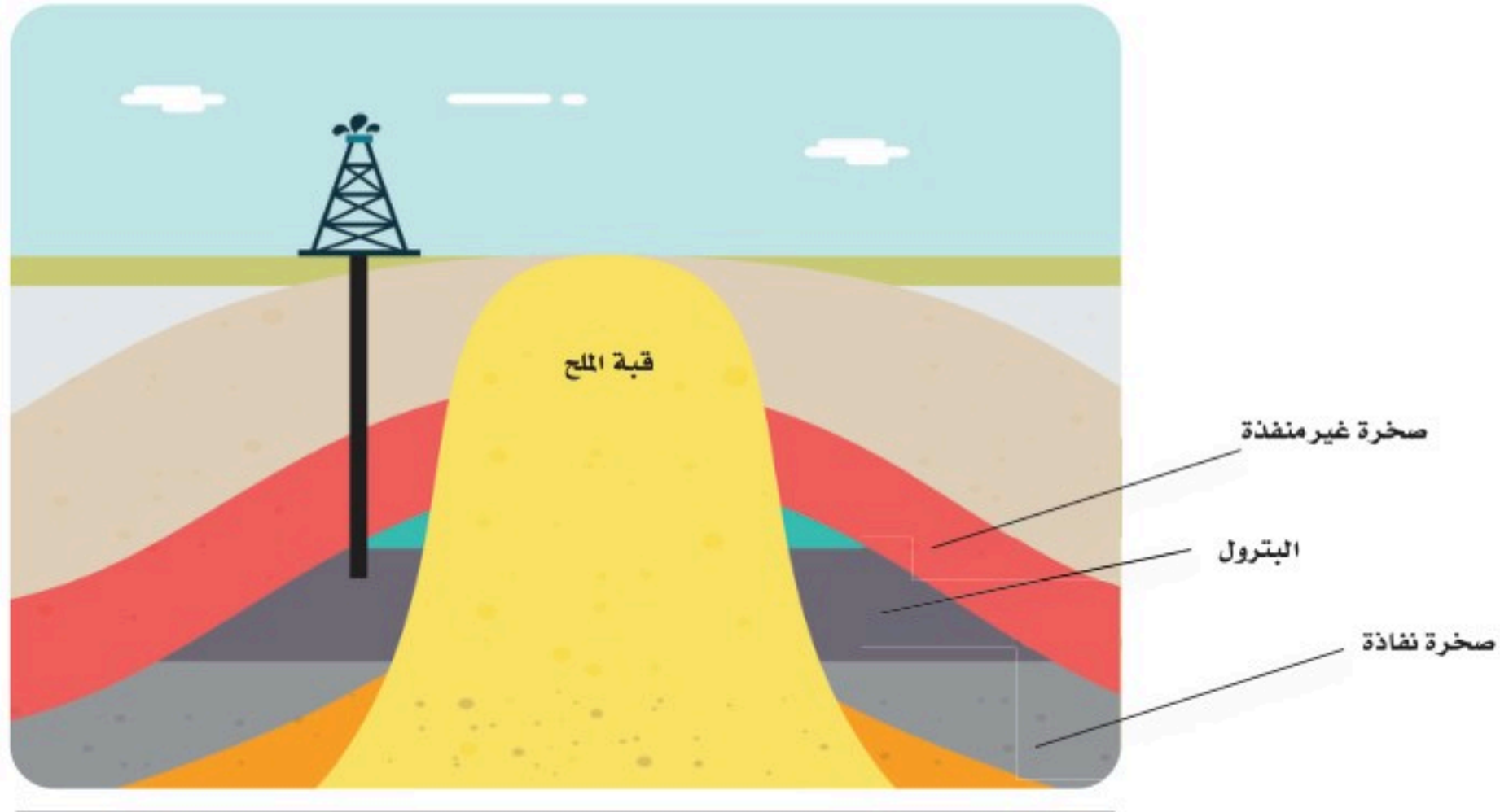
الشكل 5-5 مصائد القباب الملحية.
