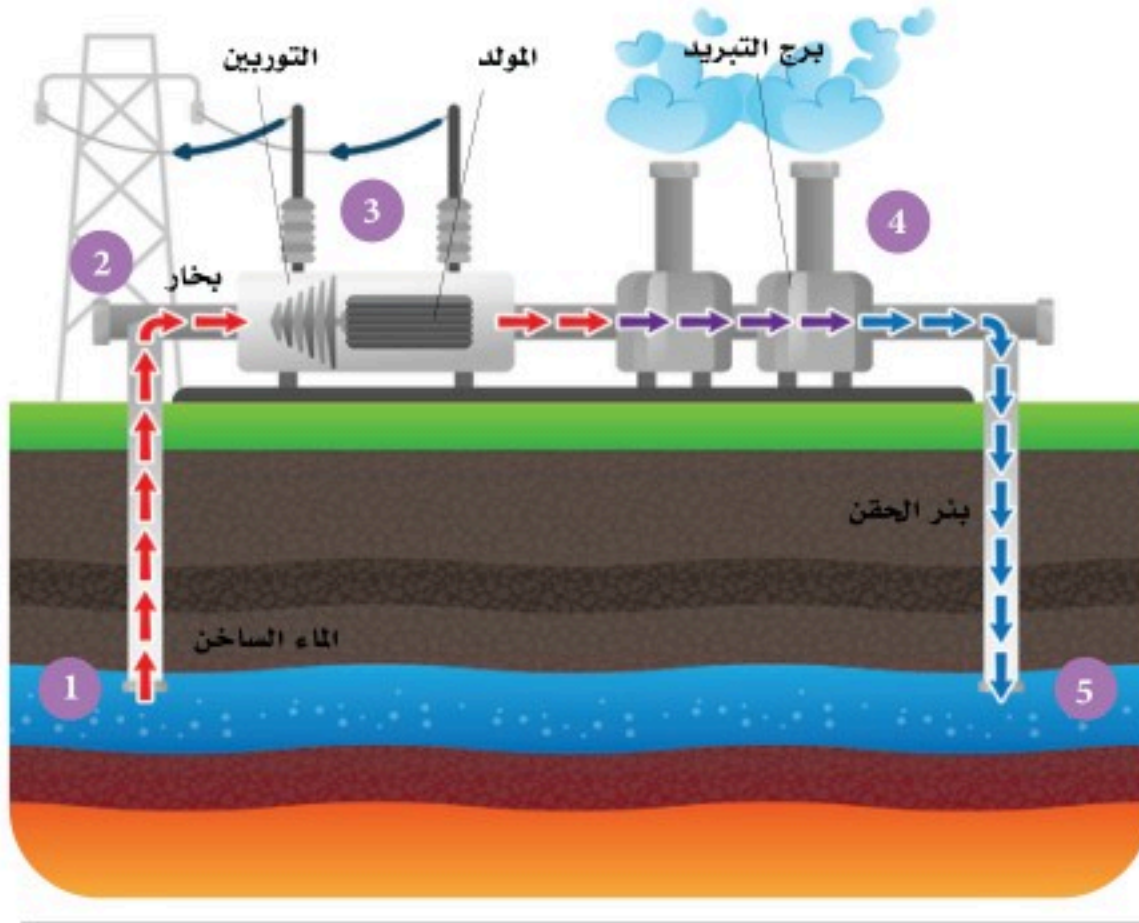
الشكل 10-5 الطاقة الحرارية الأرضية.
