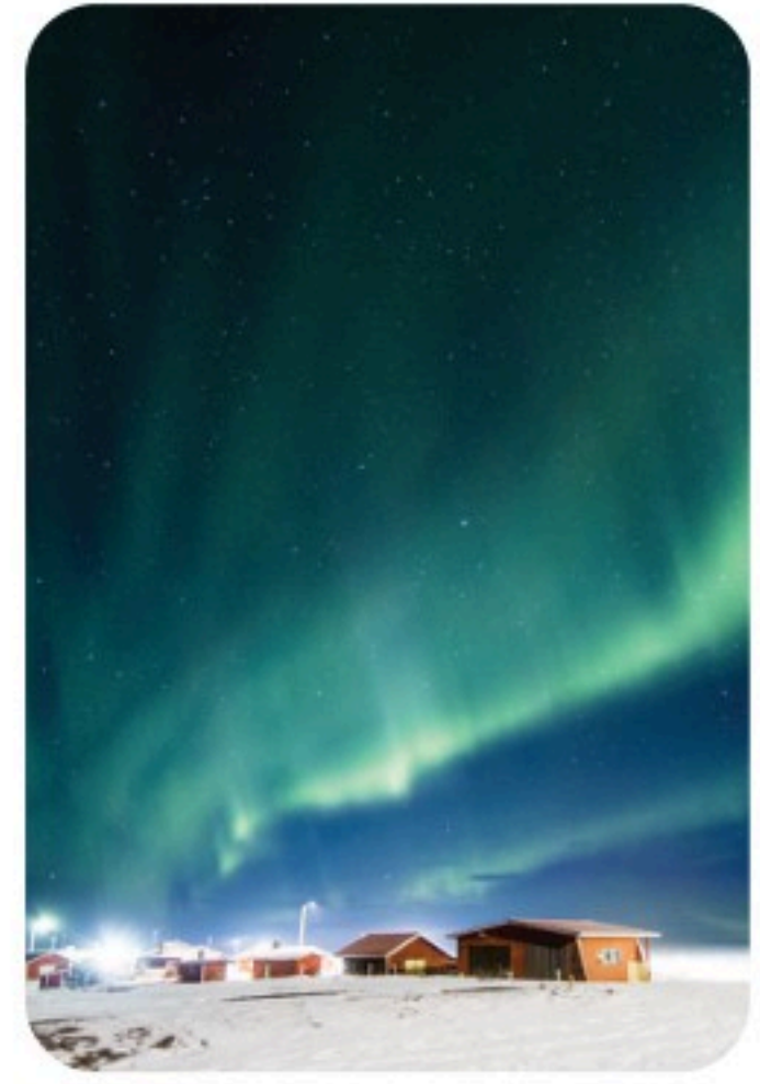
الشكل 12-2 الشفق القطبي.
