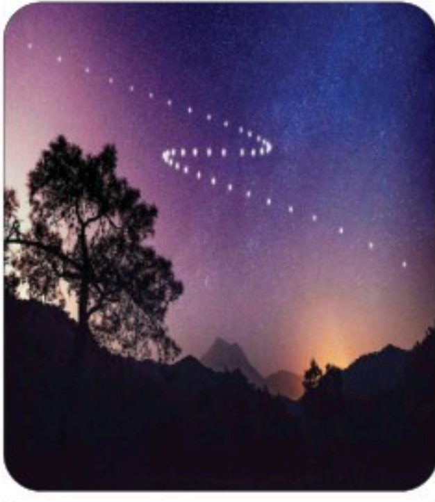
الشكل 7-1 حركة تراجعية مدارية ظاهرية لكوكب المريخ.
