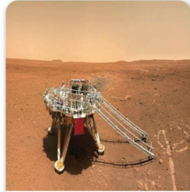
الشكل 9-1 صورة لمركبة هبوط مهمة Tianwen-1
