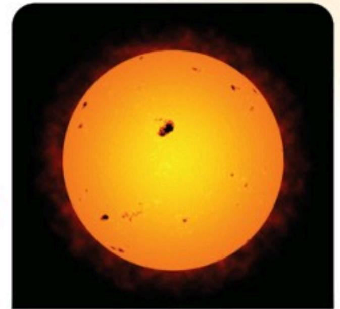
الشكل 2-8 البقع الشمسية على سطح الشمس.
