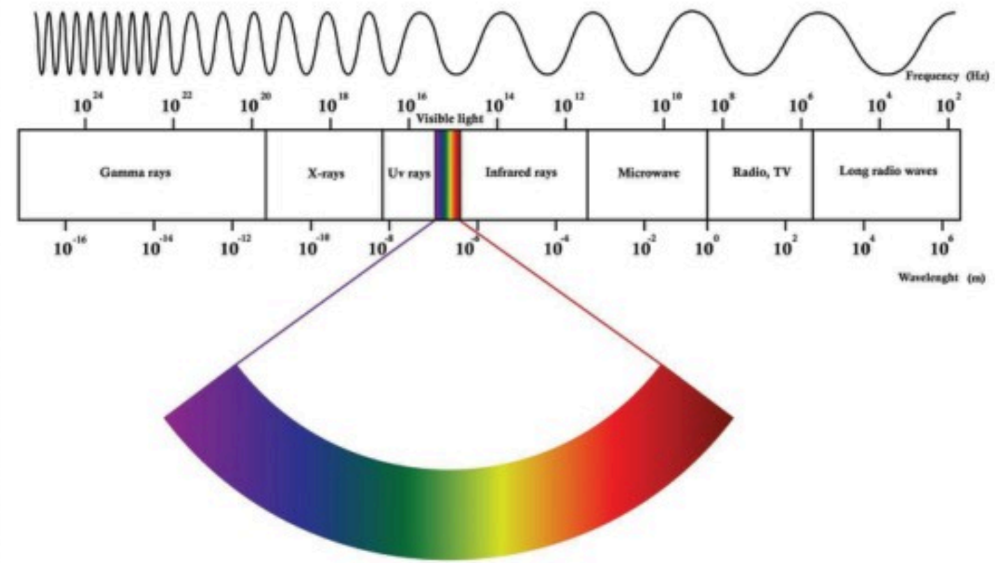
الشكل 1-3 نطاقات الطيف الكهرمغناطيسي.
