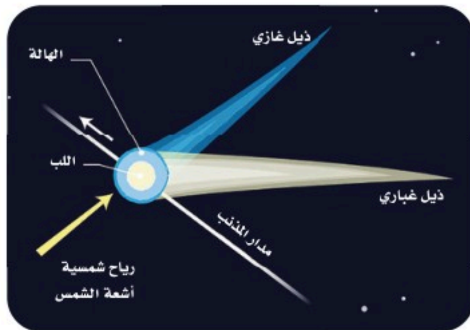
الشكل 20-1 تركيب المذنبات.
