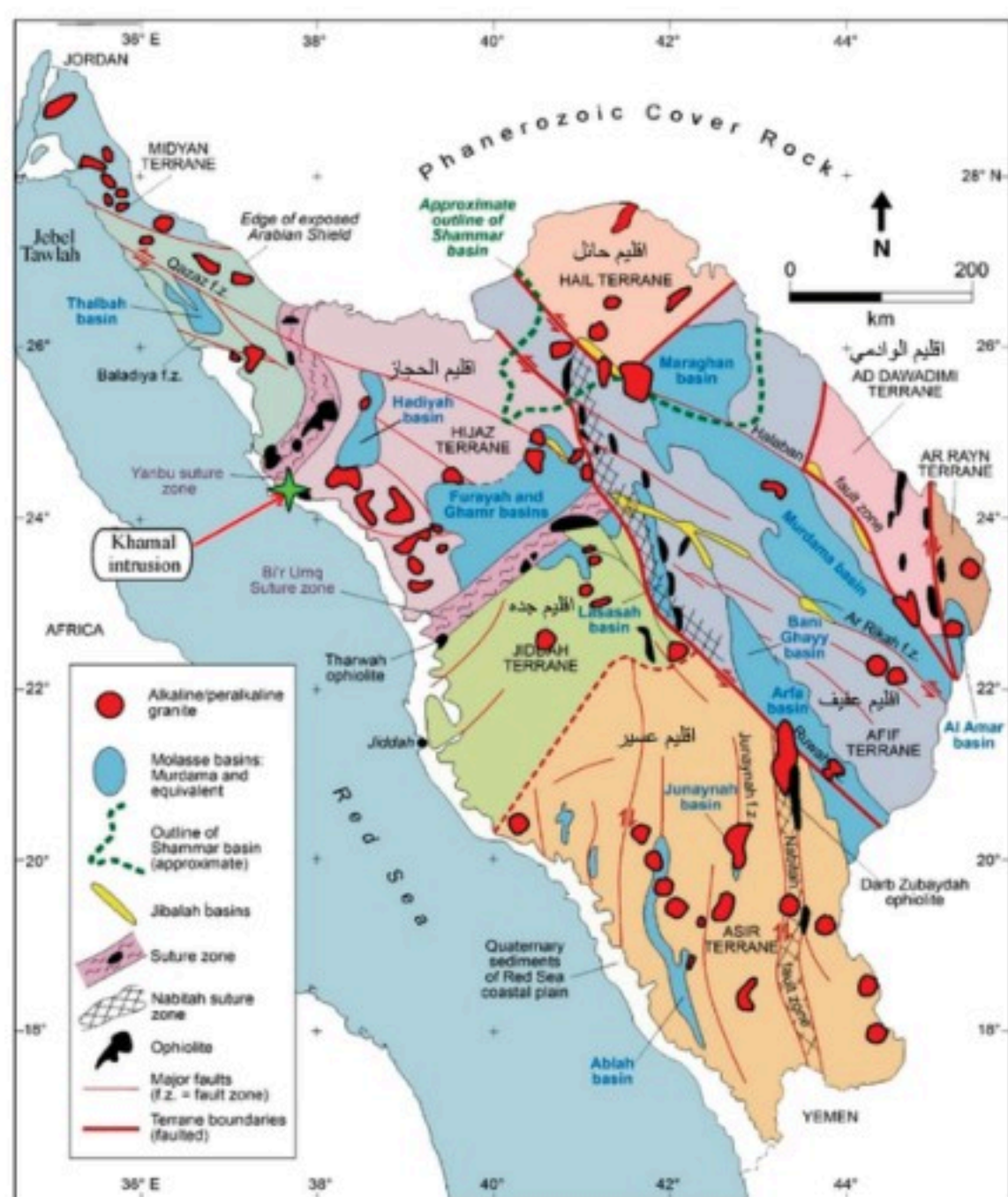
الشكل 3-6 خريطة توضح مواقع أقاليم الدرع العربي.
