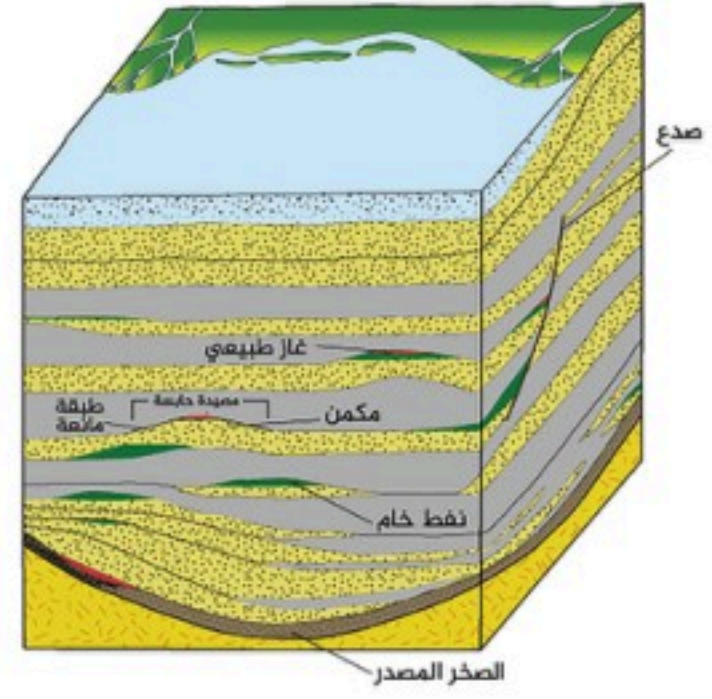
الشكل 2-5 صخر المصدر.
