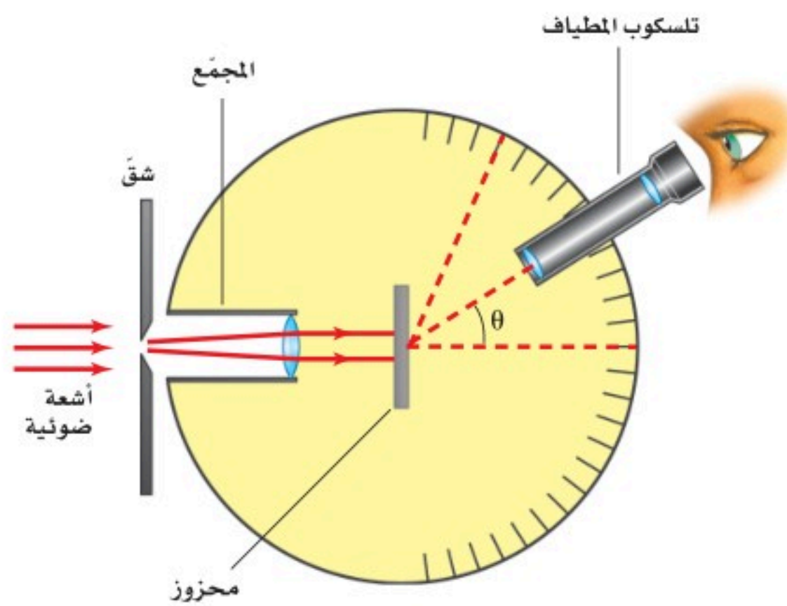
الشكل 2-3 تحليل الضوء بالمطياف.
