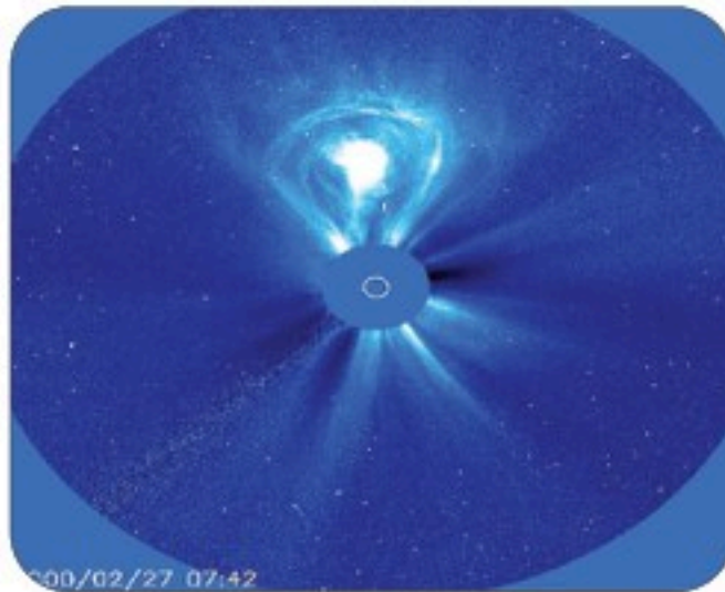
الشكل 11-2 الانبعاث الكتلي الإكليلي.
