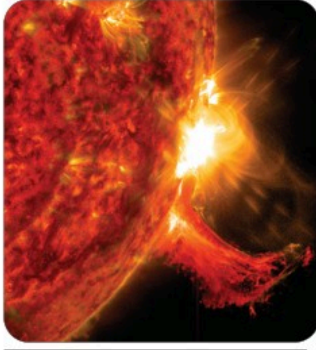
الشكل 9-2 التوهجات الشمسية.
