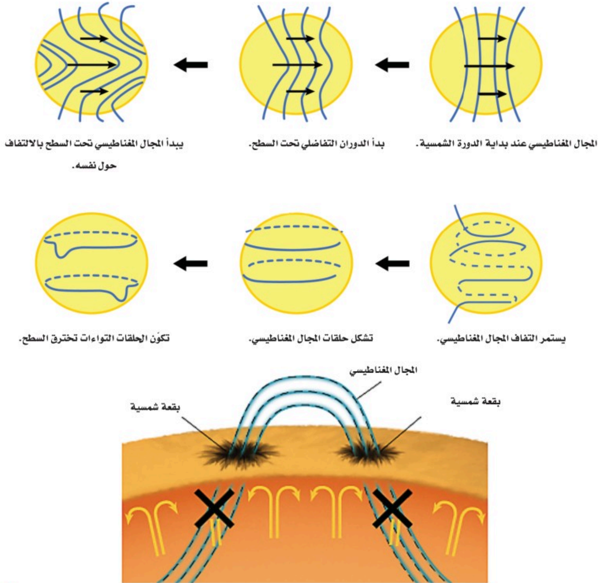
الشكل 7-2 التواء خطوط المجال المغناطيسي بسبب الدوران التفاضلي للشمس ونشوء البقع الشمسية.
