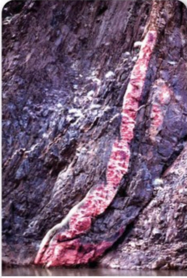
الشكل 20-4 بحسب مبدأ القاطع والمقطوع فإن القواطع النارية أحدث من صخور الشيست. استنتج كيف تكونت القواطع النارية؟
