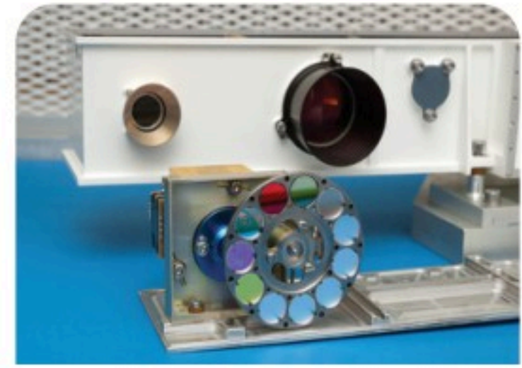
الشكل 11-3 كاميرا مثبتة بأسطوانة فلتر.
