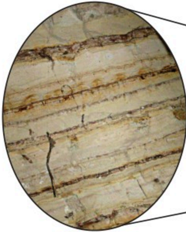
الشكل 31-4 تساعد رقائق الرسوبيات المتعاقبة العلماء على تأريخ الدورات الرسوبية في البحيرات الجليدية.
