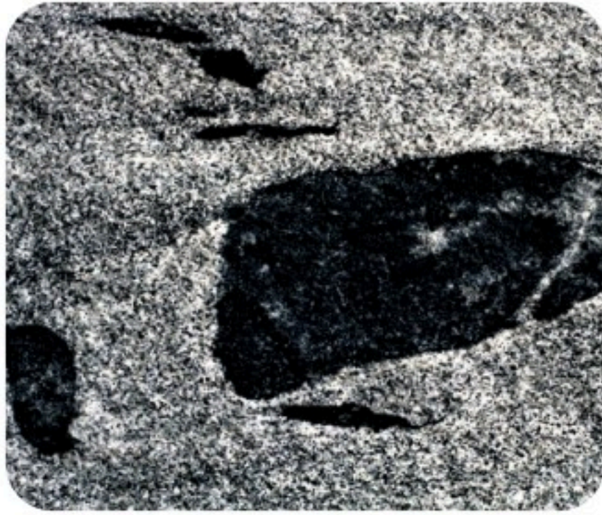
الشكل 22-4 تحتوي الصخور الحديثة على قطع صخرية من صخر قديم.
