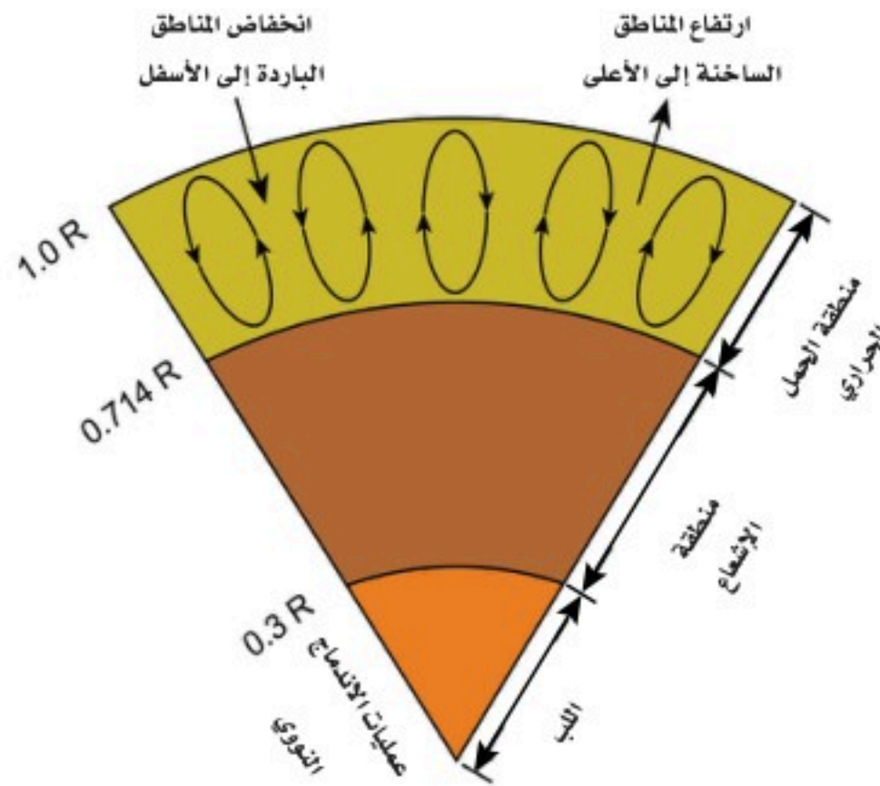
الشكل 2-3 التركيب الداخلي للشمس.
