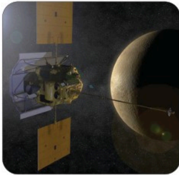
الشكل 5-1 صورة لمركبة ميسنجر.
