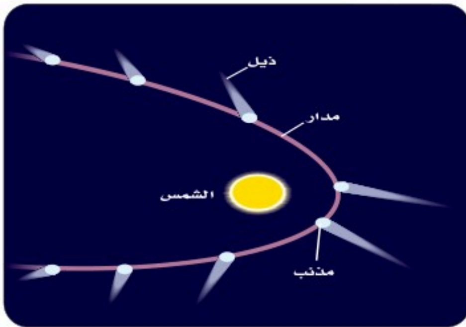
الشكل 19-1 مدار المذنبات واتجاه ذيل المذنب عند اقترابه من الشمس.
