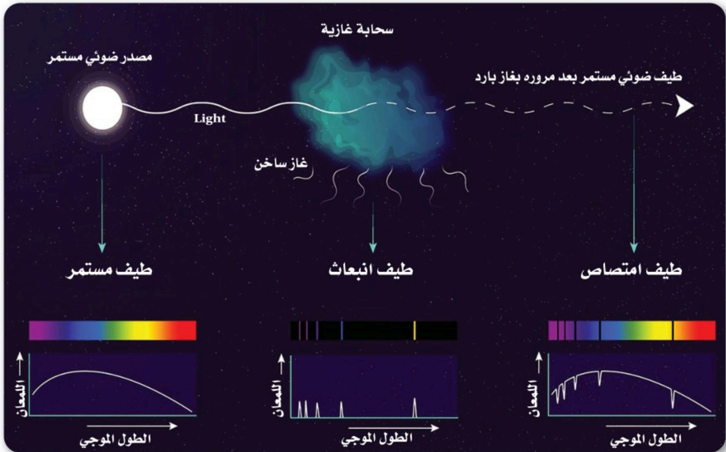
الشكل 3-3 الفرق بين طيف الانبعاث وطيف الامتصاص والطيف المستمر.
