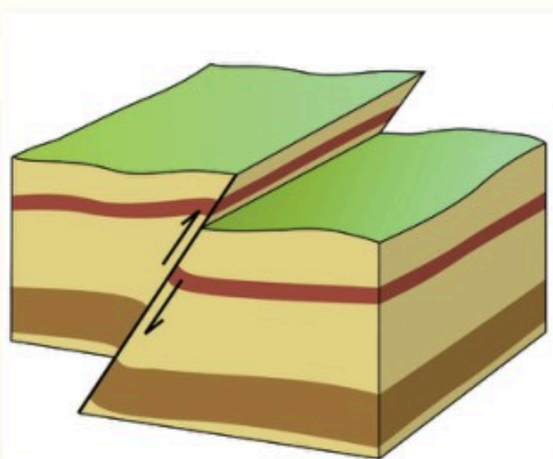
نموذج لمكمن صدعي.
