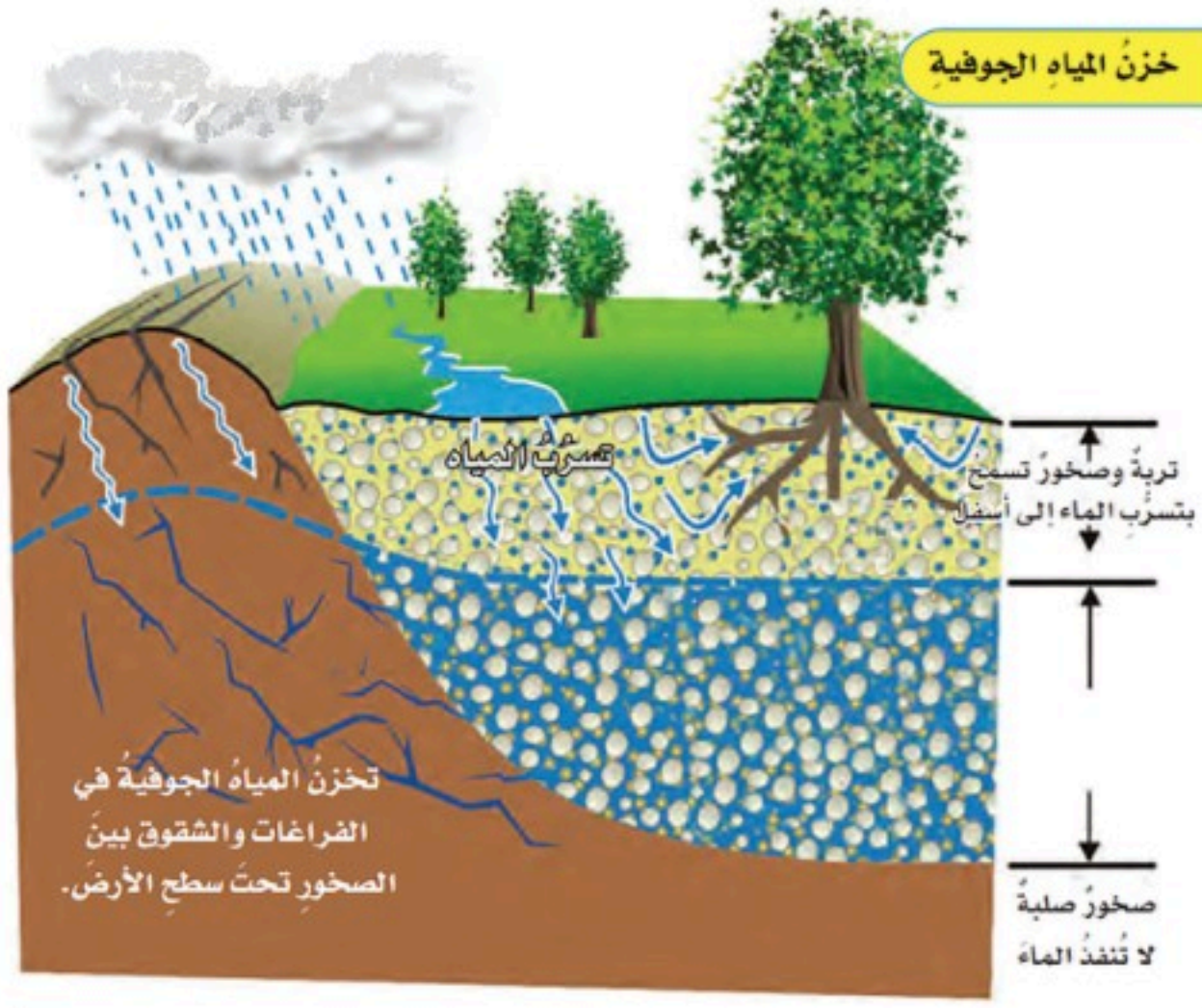
الشكل 15-6 تخزين المياه الجوفية.
