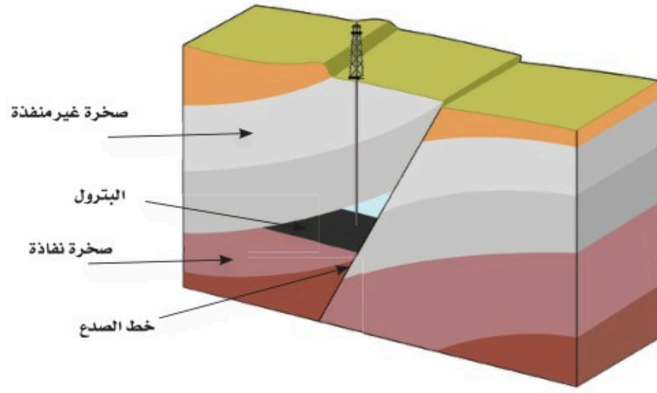
الشكل 4-5 مصادد الصدوع.
