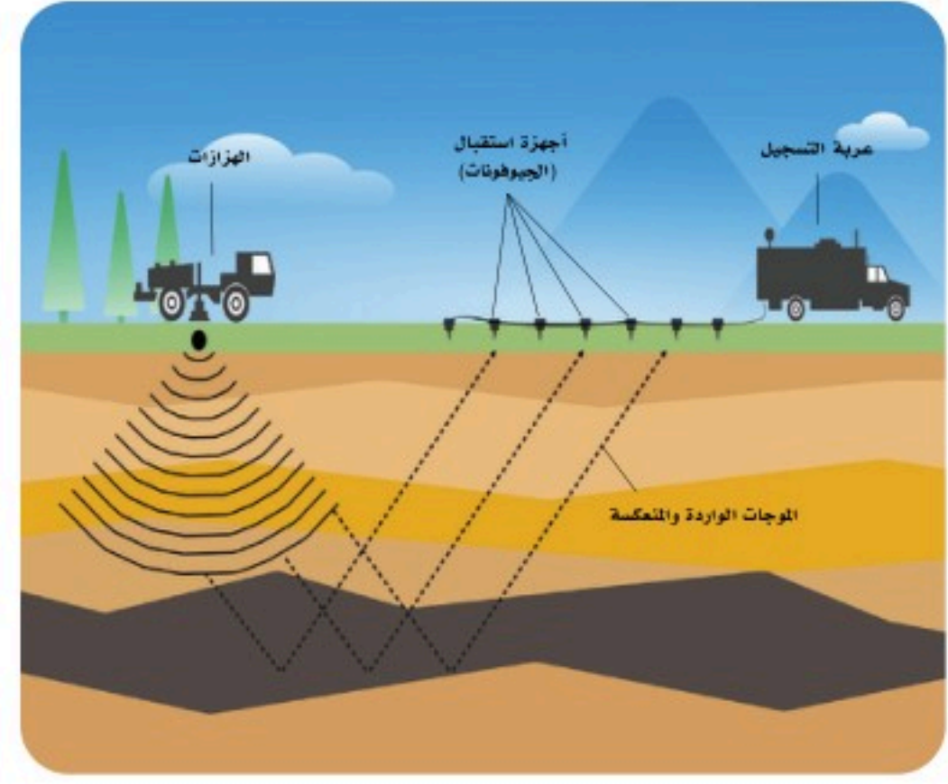
الشكل 5-7 المسح الزلزالي.
