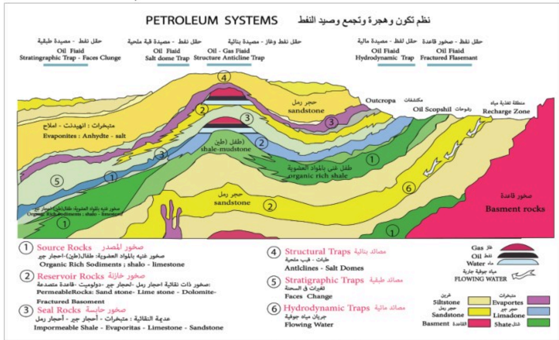
الشكل 1-5 النظام النفطي.
