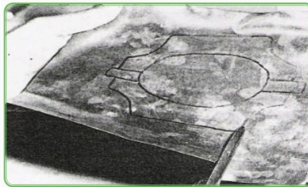
الشكل (٧٨): قص النحاس.
