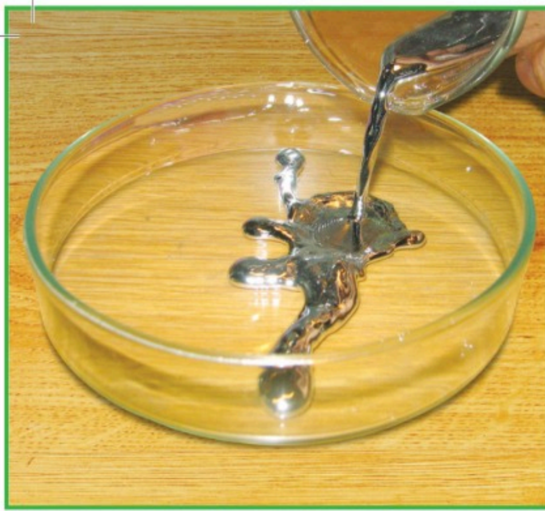
الزئبق فلز في الحالة السائلة
