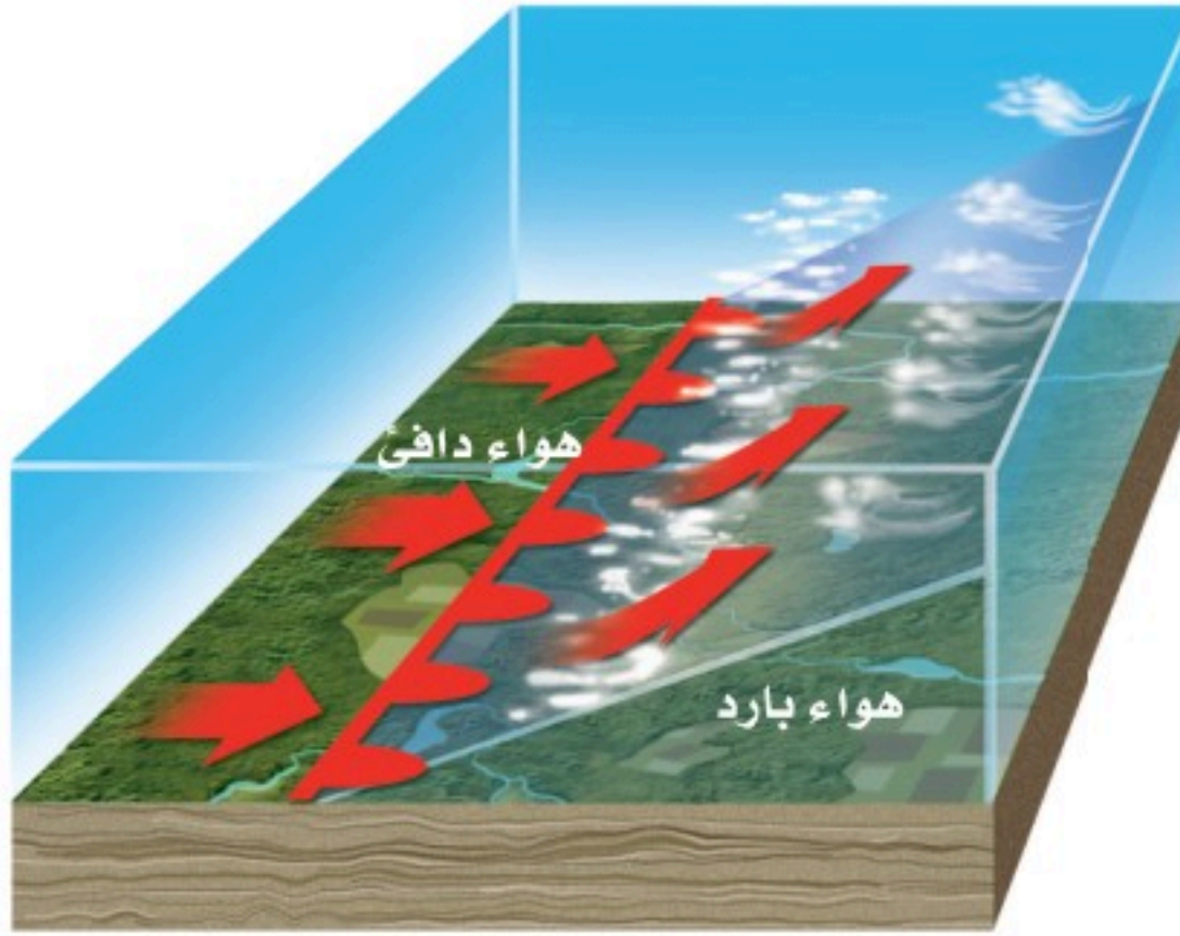
تشكل جبهة دافئة
