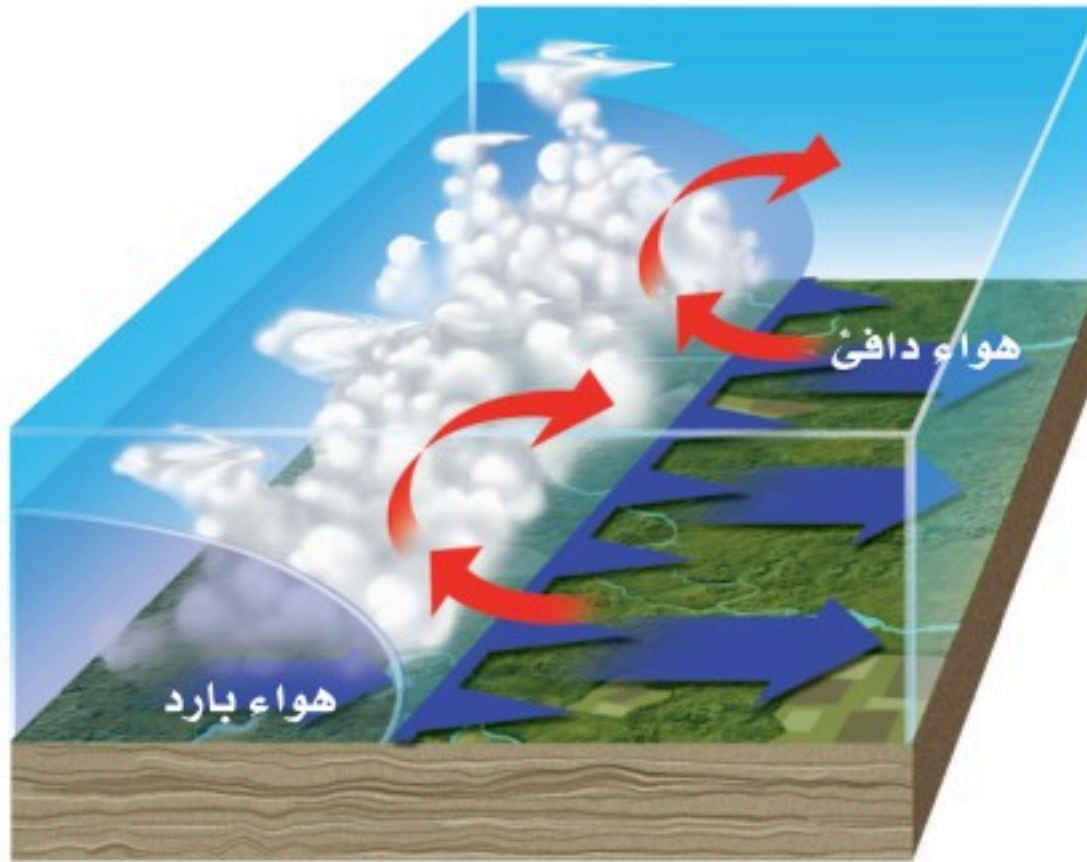
تشكل جبهة باردة
