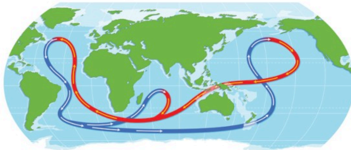
شكل 8-19 انتقال الحرارة عبر تيارات المحيطات.
