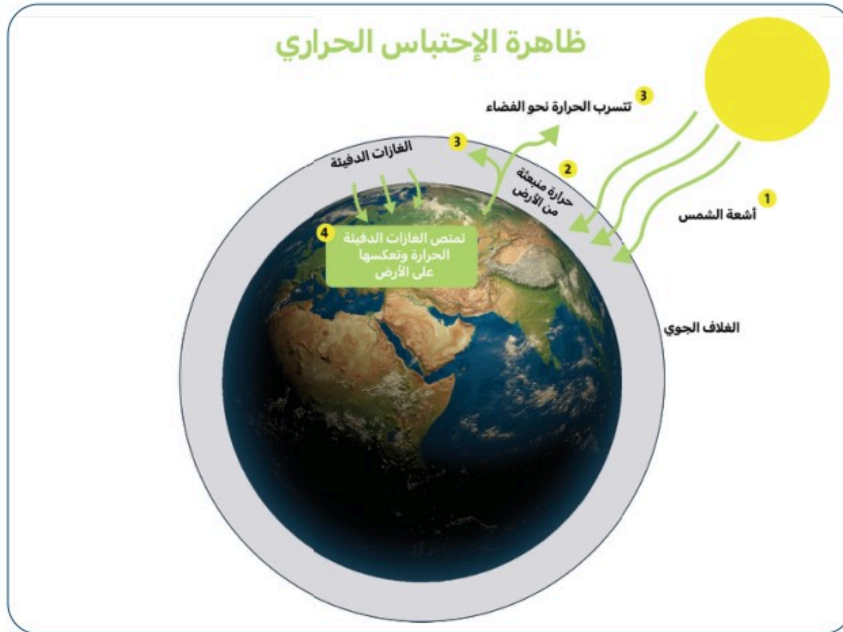
شكل 2-9 ظاهرة الإحتباس الحراري.
