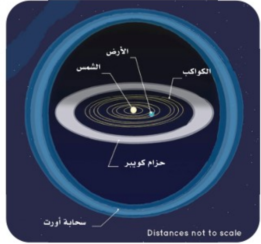
الشكل 21-1 مدار المذنبات قصيرة المدى وطويلة المدى. المصدر: وكالة ناسا.
