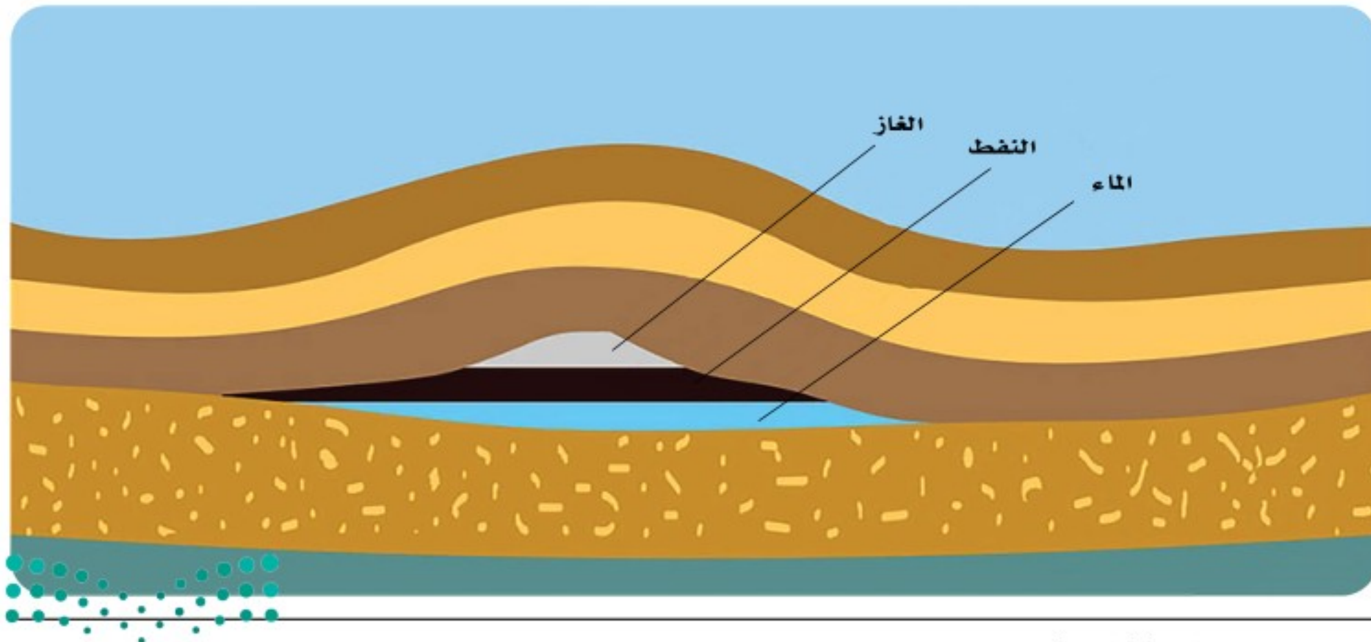
الشكل 3-5 مصائد الطيات المحدبة.
