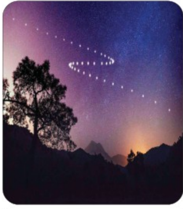
الشكل 7-1 حركة تراجمية مدارية ظاهرية لكوكب المريخ.
