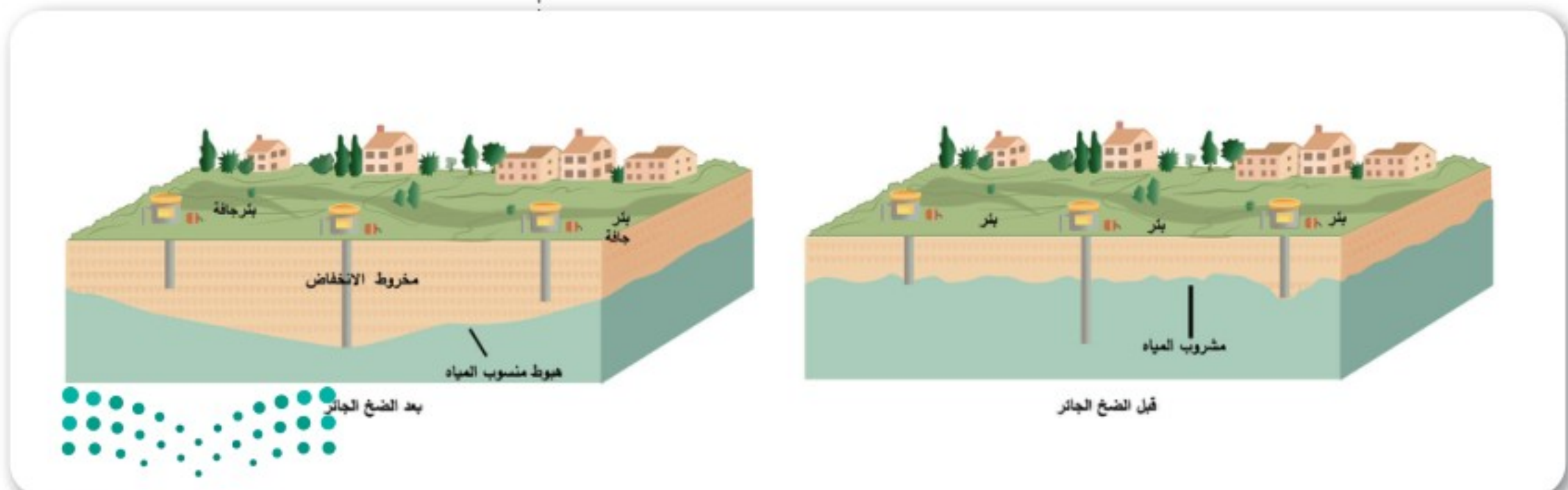
الشكل 18-6 تأثير الضخ الجائر على المياه الجوفية.
