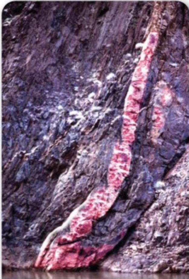
الشكل 4-20 بحسب مبدأ القاطع والمقطع فإن القواطع النارية أحدث من صخور الشيست.
