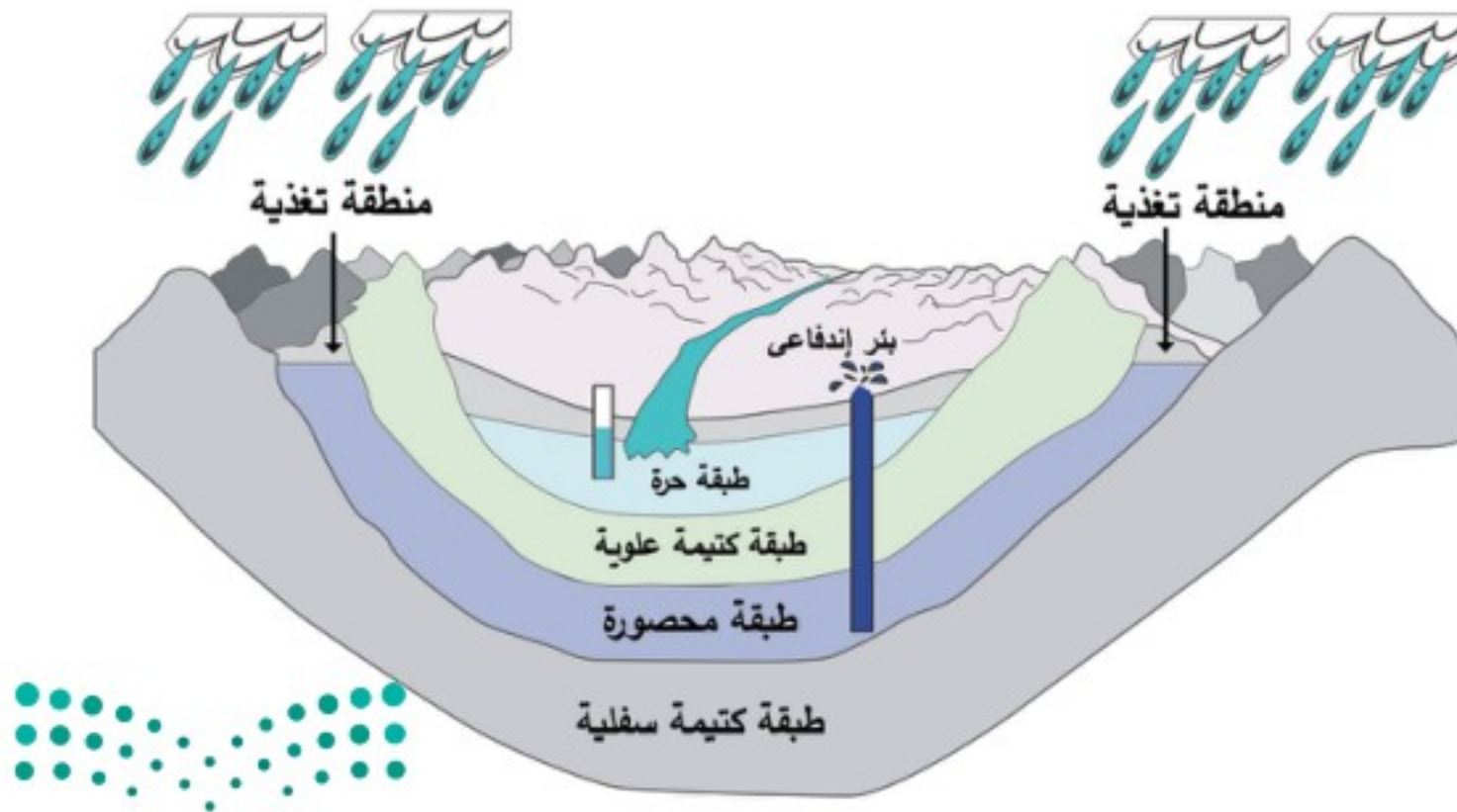
الشكل 16-6 الطبقة المحصورة.
