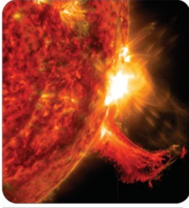
الشكل 9-2 التوهجات الشمسية.
