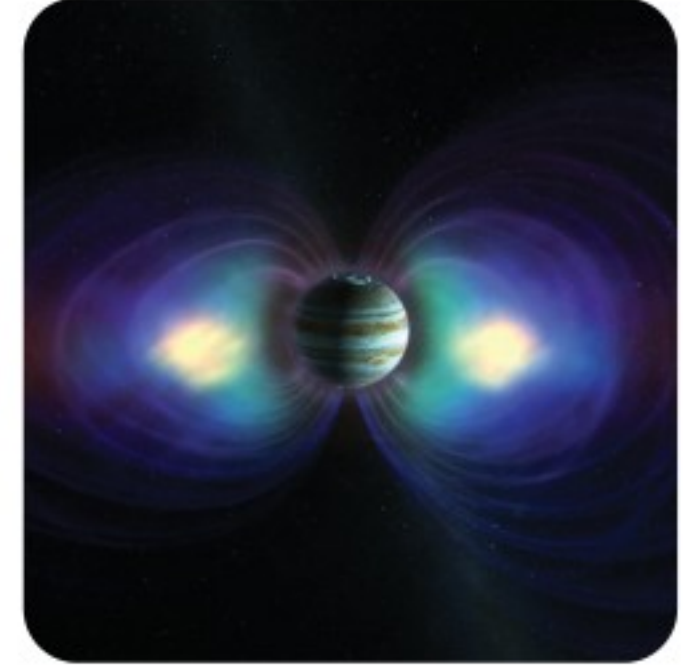
الشكل 15-3 المجال المغناطيسي للمشتري.
