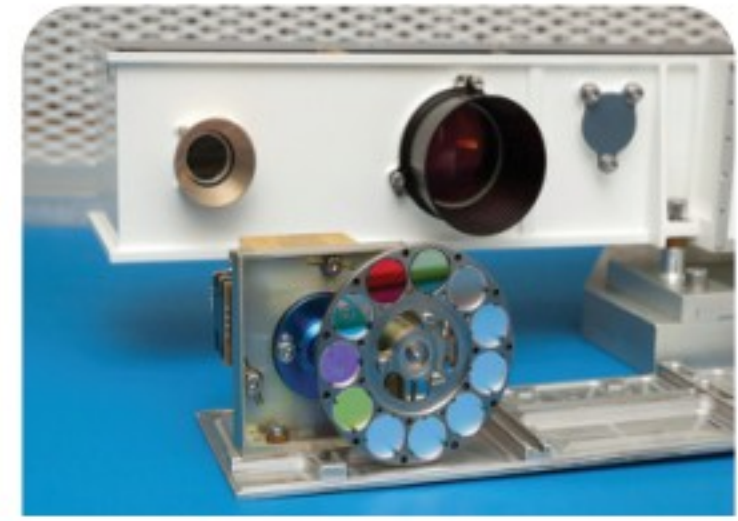
الشكل 11-3 كاميرا مثبتة بأسطوانة فلاتر.
