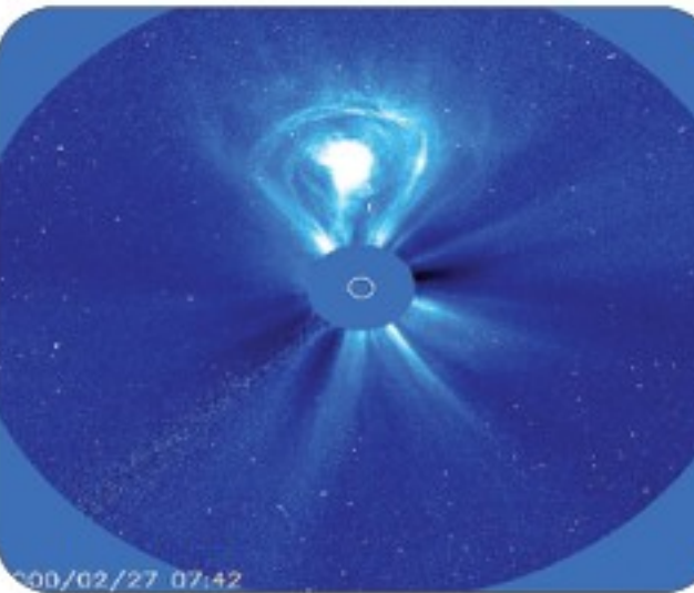
الشكل 11-2 الانبعاث الكتلي الإكليلي
