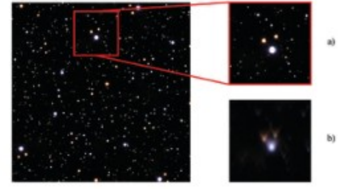
الشكل 10-3 صورة توضح الزيغ الهالي.
