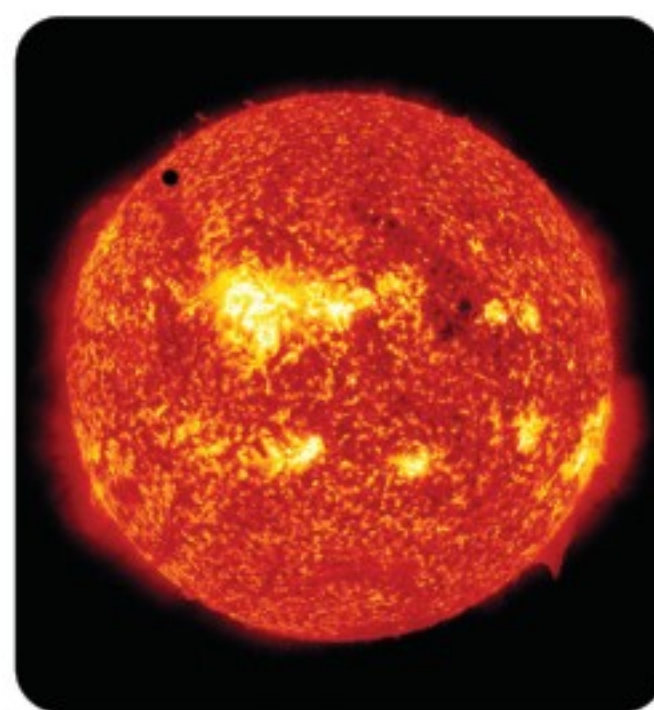
الشكل 2-4 طبقة الغلاف الضوئي وتظهر الحبيبات في السطح.
