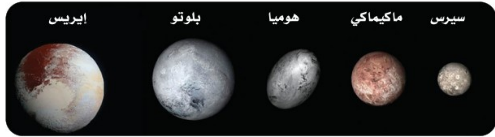
الشكل 2-1 الكواكب القزمة في نظامنا الشمسي.
