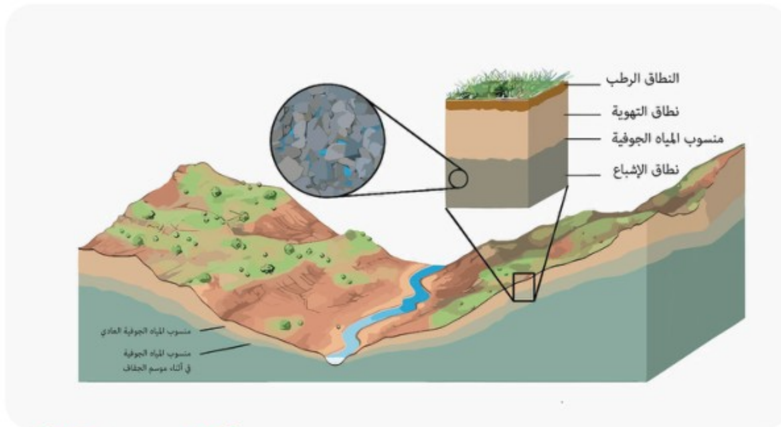
الشكل 14-6 المياه الجوفية.
