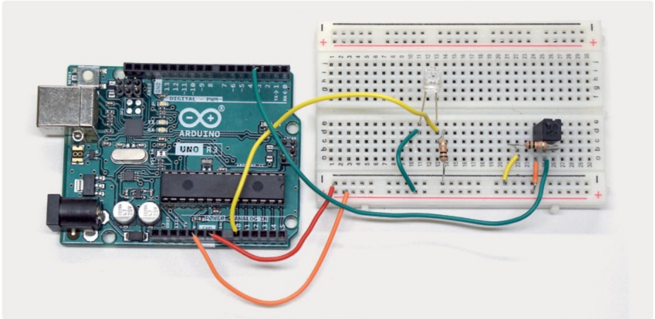
شكل 7.17: صورة للدائرة
