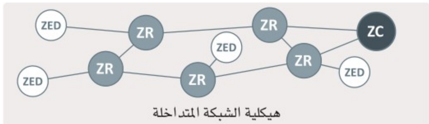
شكل 5.23: هيكليات زيجبي
