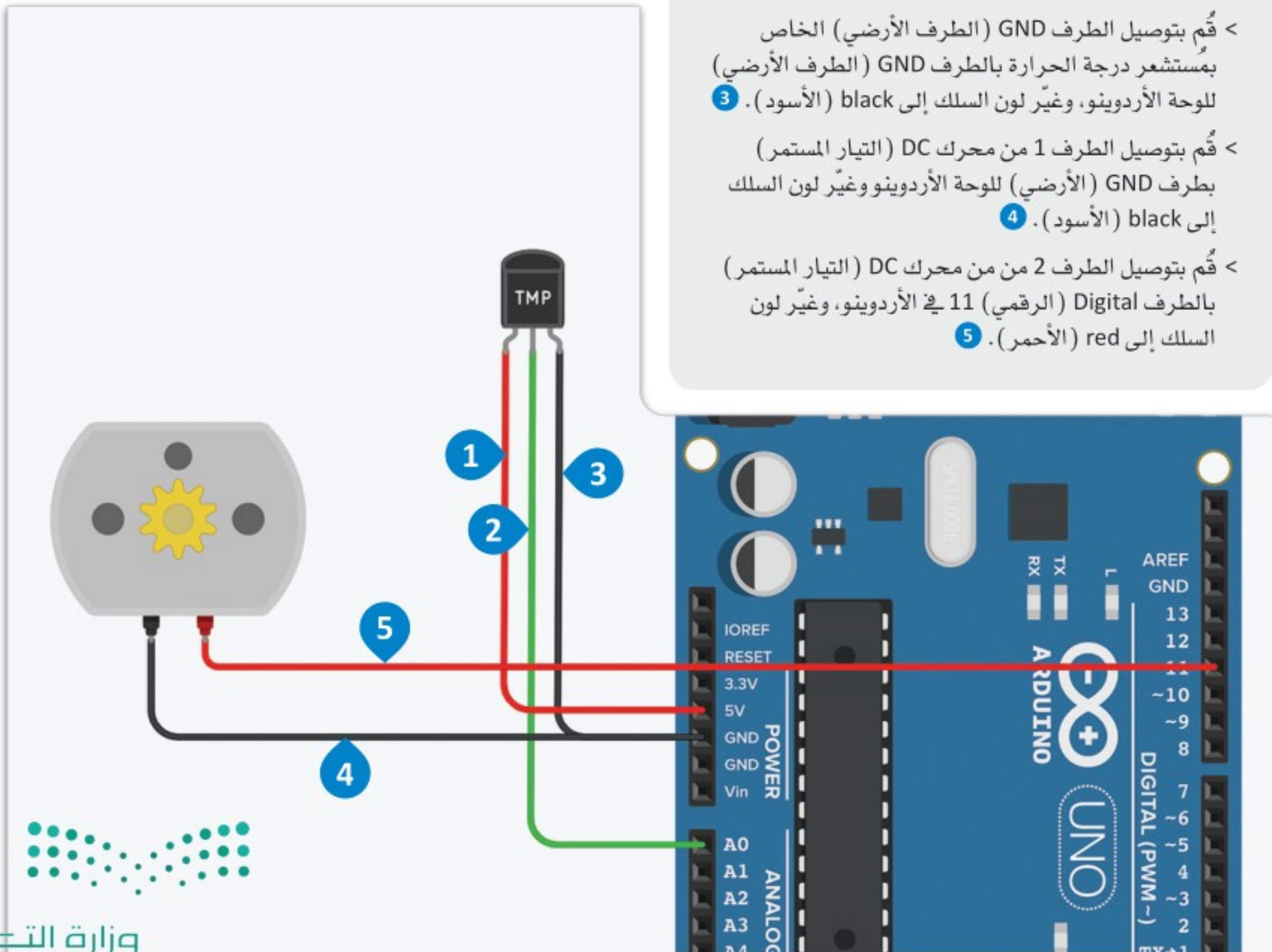
شكل 6.16: توصيل الدائرة
