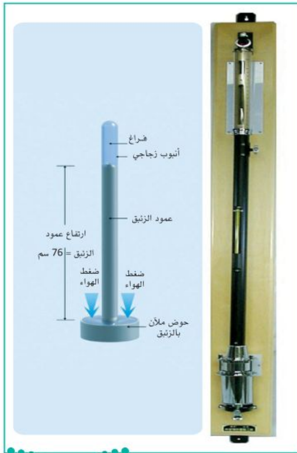
البارومتر الزئبقي
