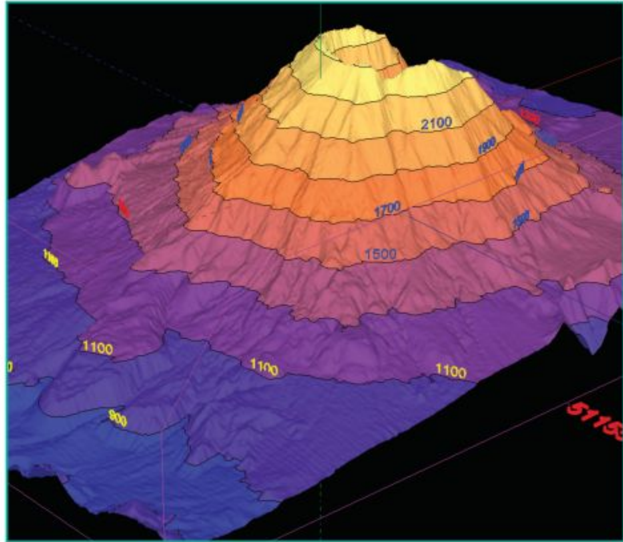
خطوط الكُنْتُور
