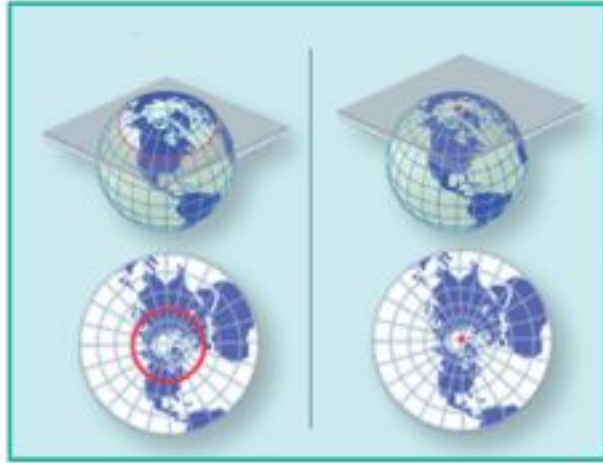
المسقط المستوي
