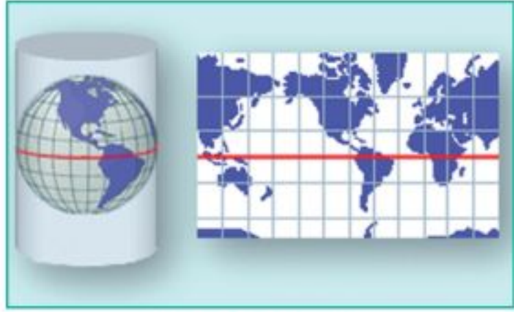
المسقط الأسطواناني
