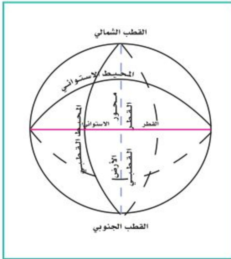
أبعاد الأرض
