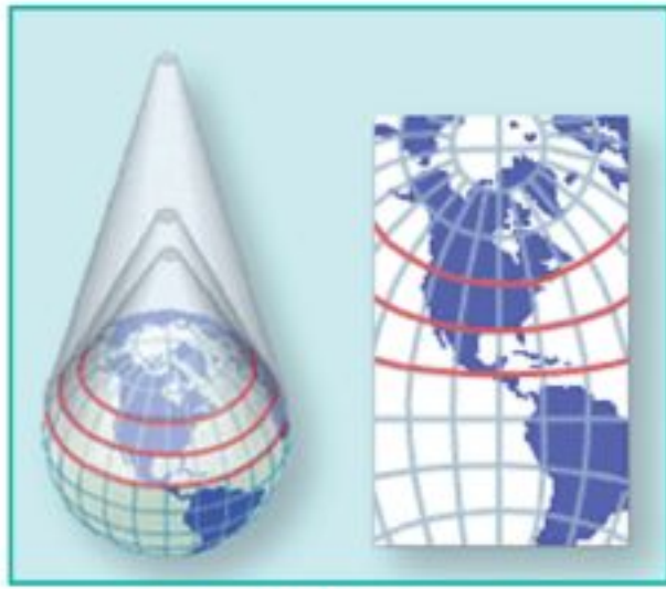
المسقط المخروطي
