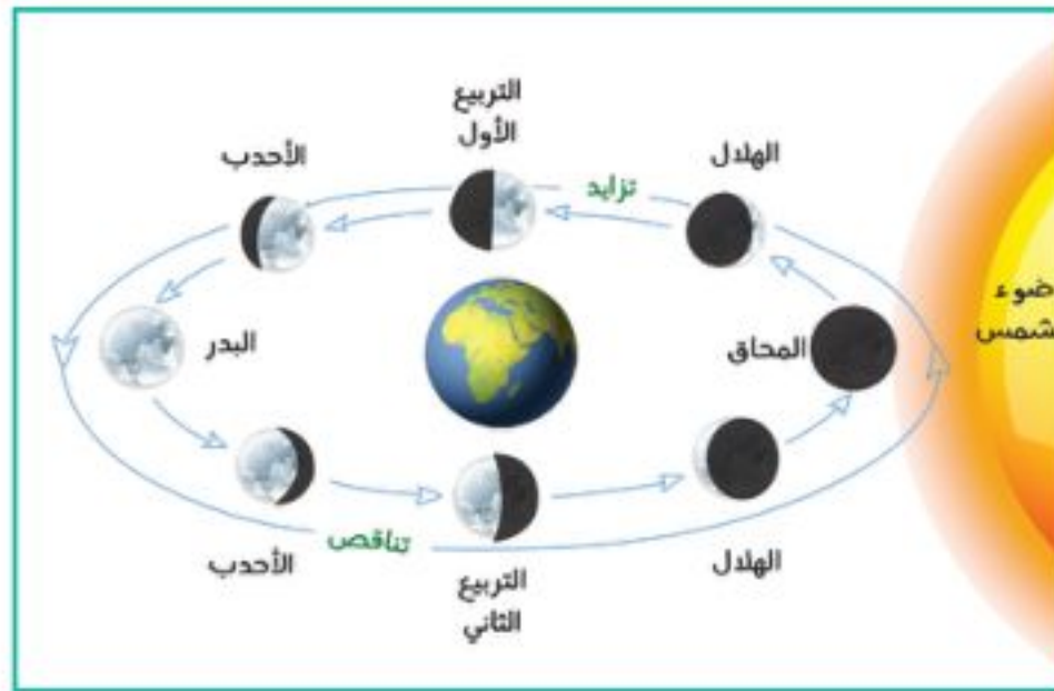
أوجه القمر
