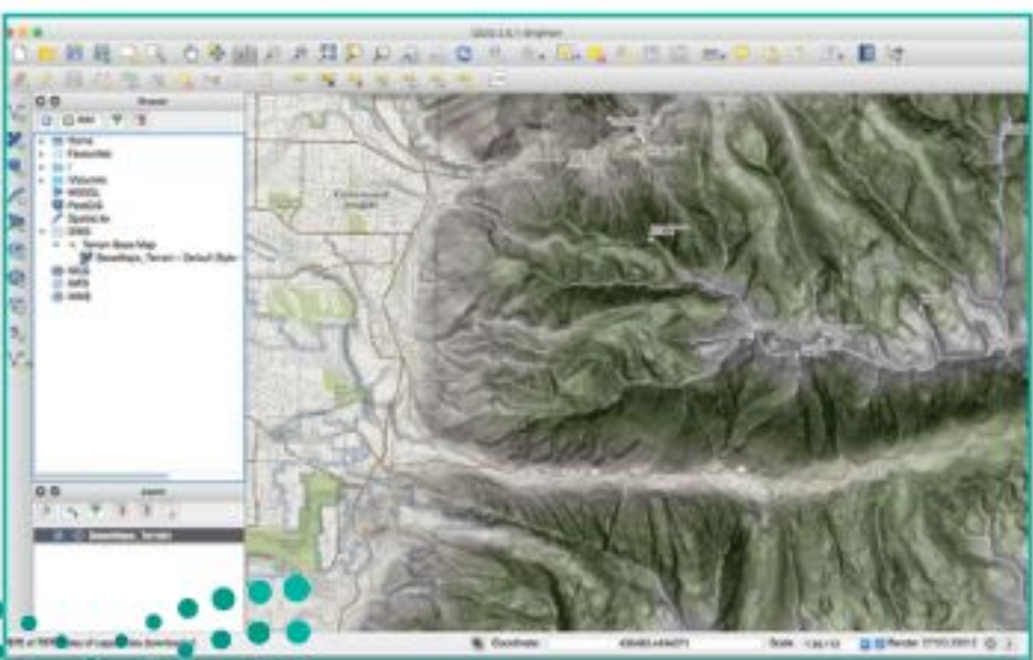
برنامج QGIS
