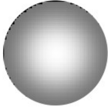
نموذج دالتون للذرة
